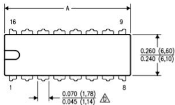
DIP16
