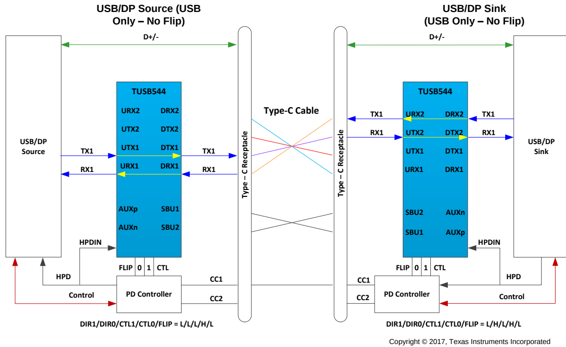
图 37. USB3.1 Only – No Flip
