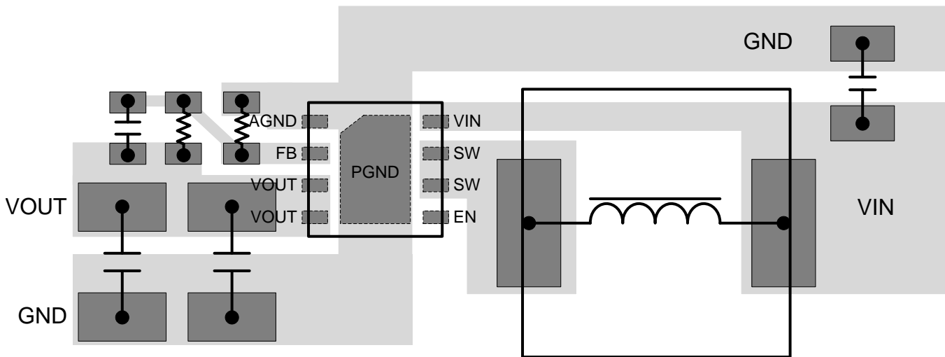
图 18. Layout Example
