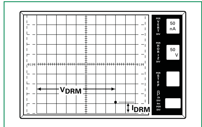
Figure AN1006.18 (+) I_{DRM} = 51 nA at (+) V_{DRM} = 400 V
