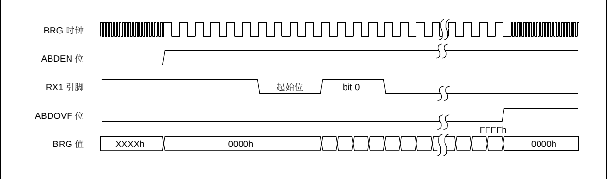
图 18-2: BRG 溢出序列
