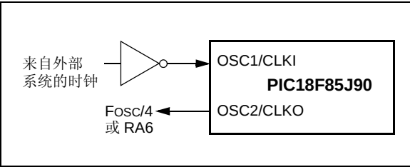
图 3-3: 外部时钟输入工作原理 (EC 配置)
