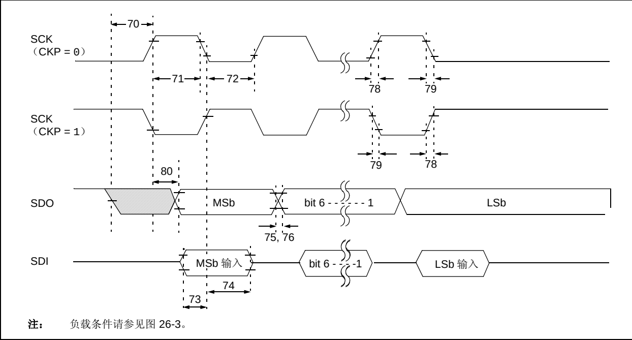
图 26-9: SPI 主控模式时序示例 (CKE = 0)
