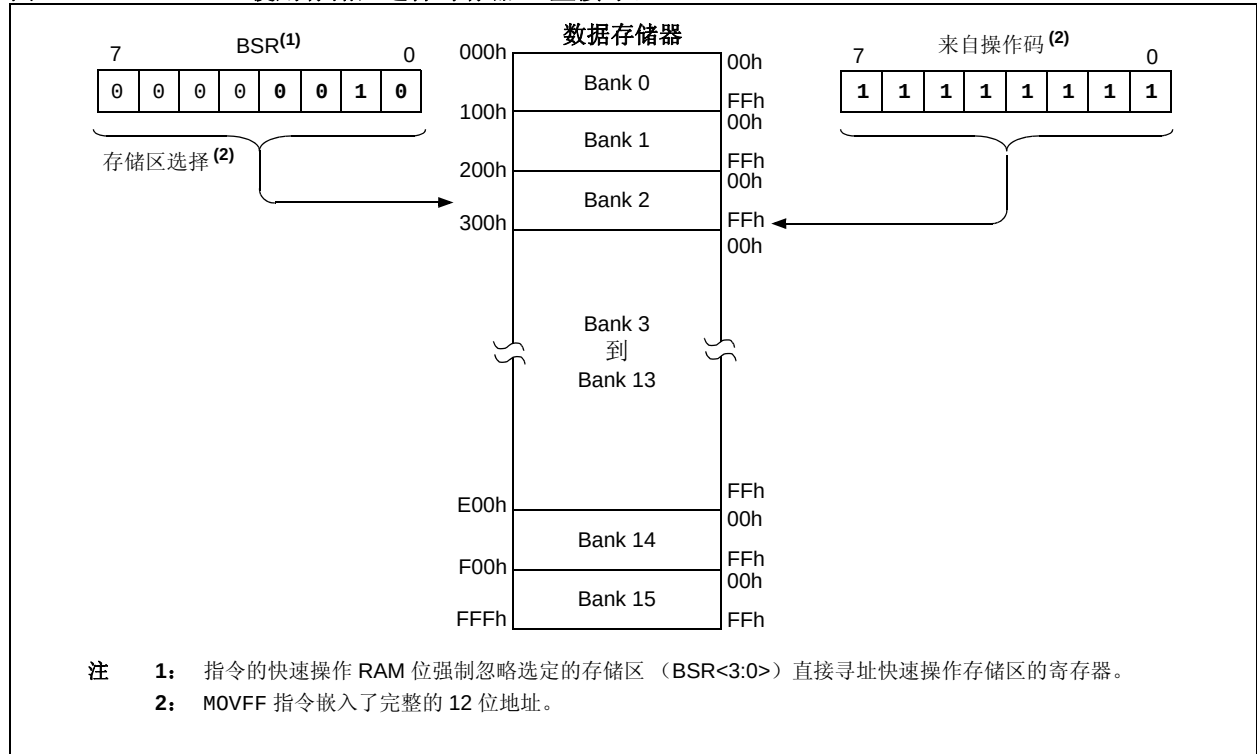
图 6-8: 使用存储区选择寄存器（直接寻址）
