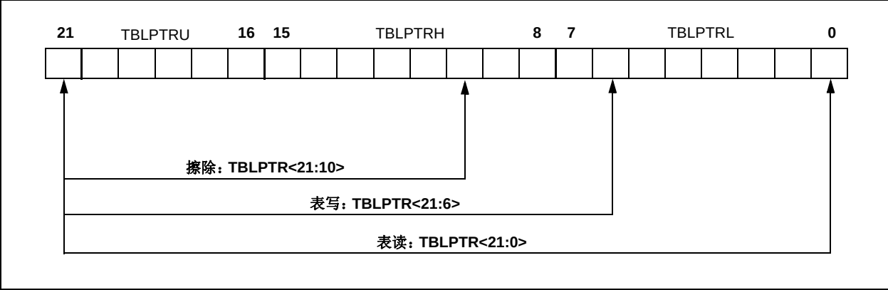
图 7-3: 基于操作的表指针范围
