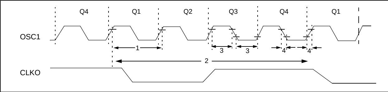
图 26-4: 外部时钟时序（除 PLL 外的所有模式）
