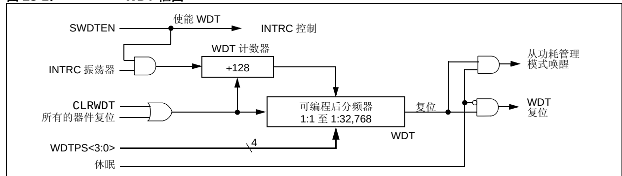
图 23-1: WDT 框图
