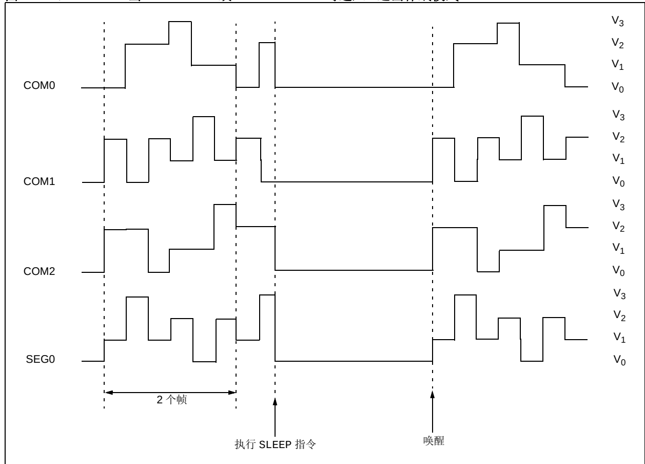
图 16-18: 当 SLPEN = 1 或 CS<1:0> = 00 时进入 / 退出休眠模式
