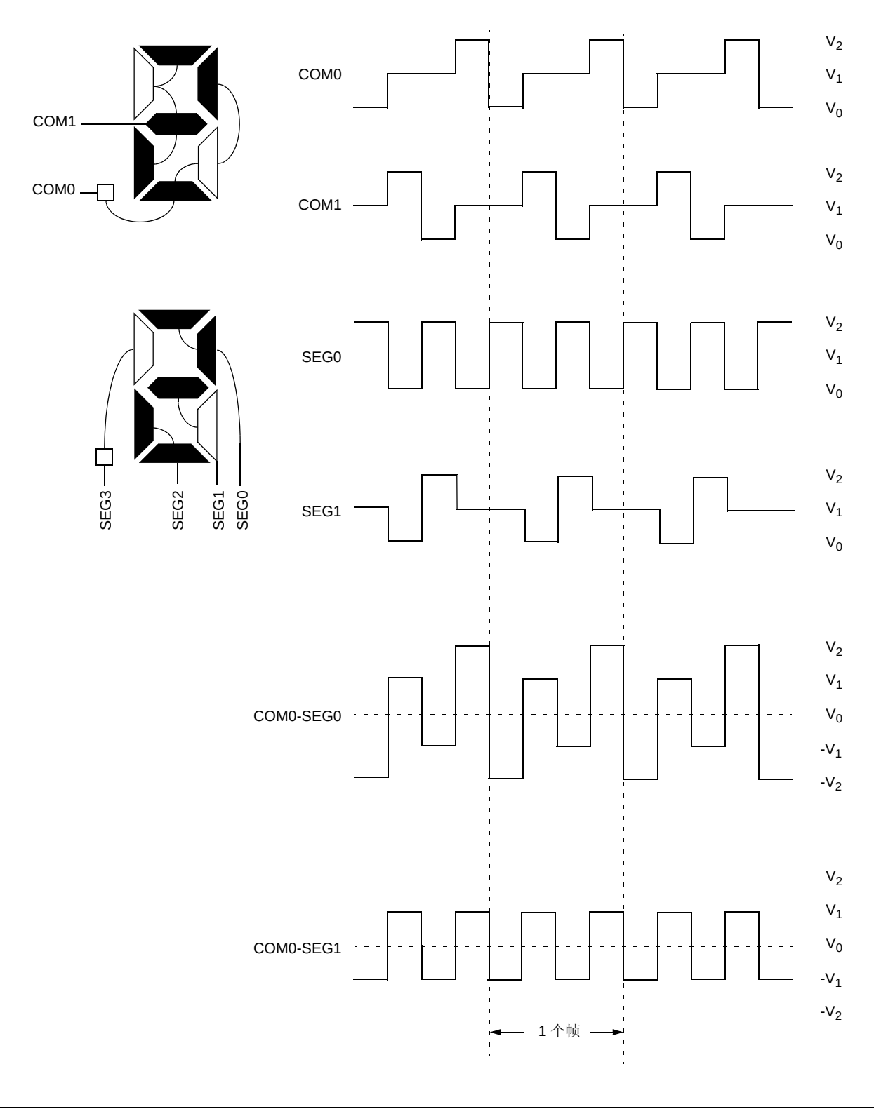
图 16-7: 在 1/2 复用、1/2 偏置驱动时的 A 型波形
