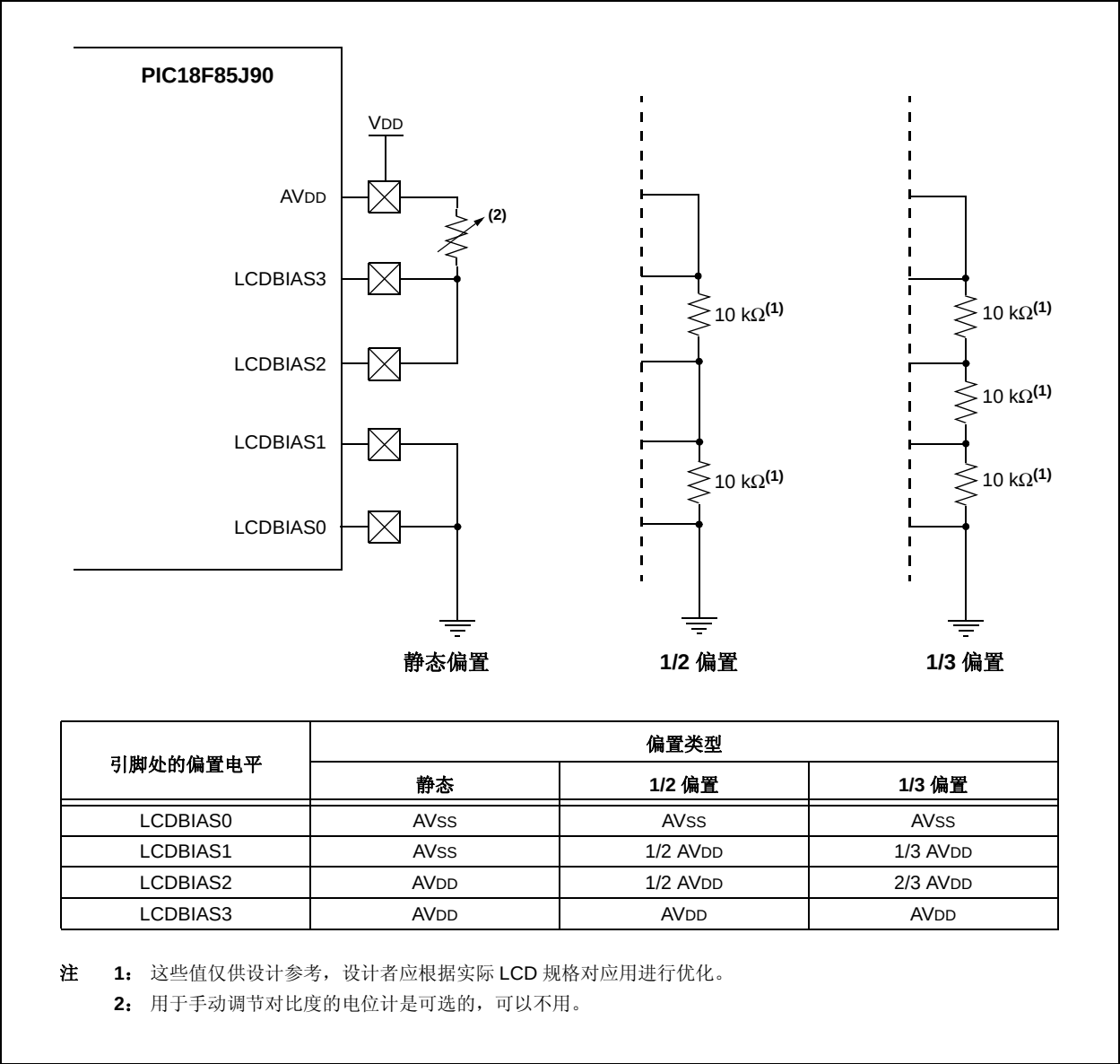
图 16-5: M3 配置的电阻梯形网络连接
