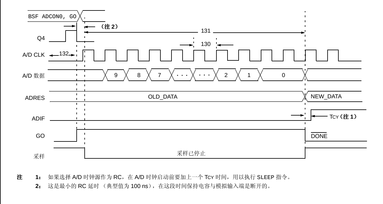
图 26-19: A/D 转换时序
