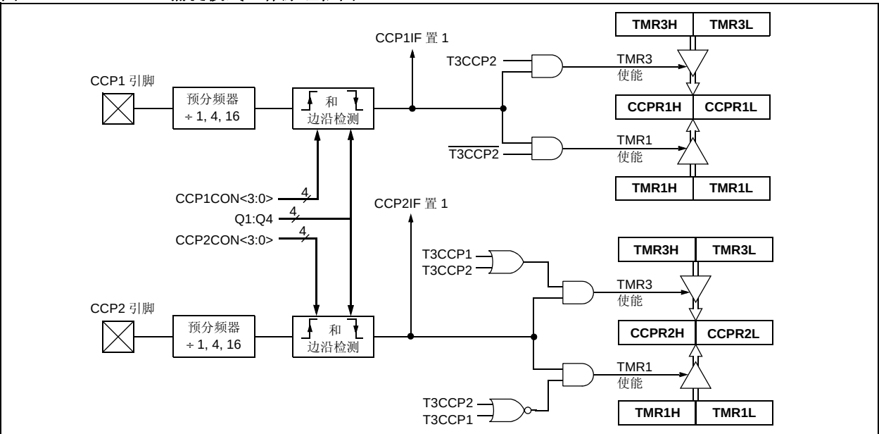
图 15-2: 捕捉模式工作原理框图
