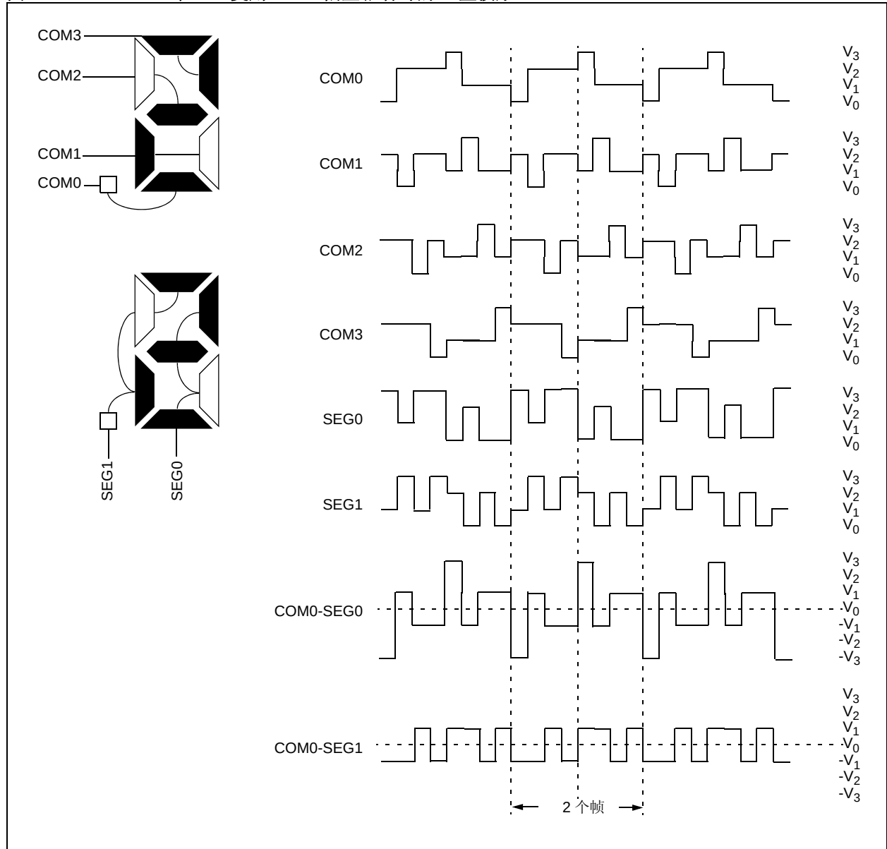
图 16-16: 在 1/4 复用、1/3 偏置驱动时的 B 型波形
