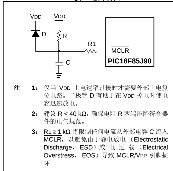
图 5-2: 外部上电复位电路（ V_{DD} 缓慢上电的情况）
