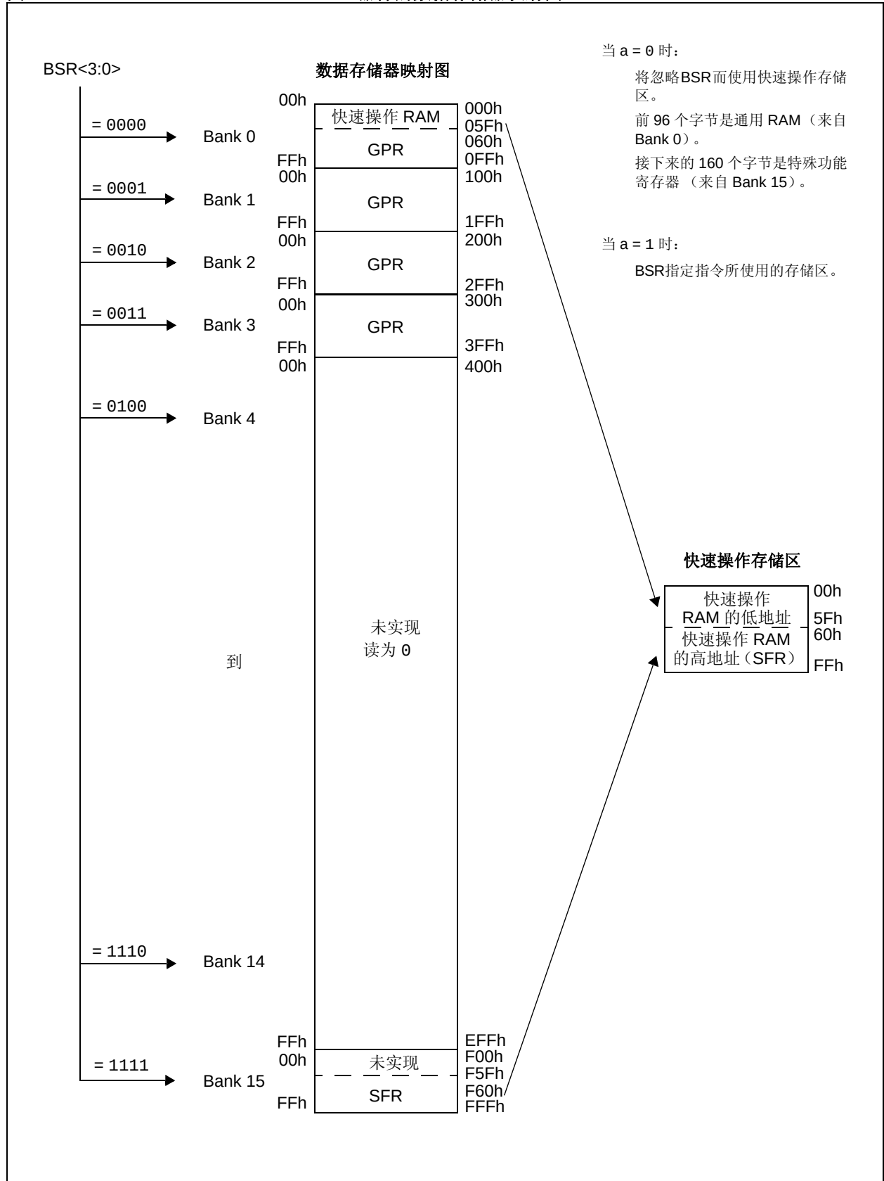
图 6-6: PIC18FX3J90/X4J90 器件的数据存储器映射图
