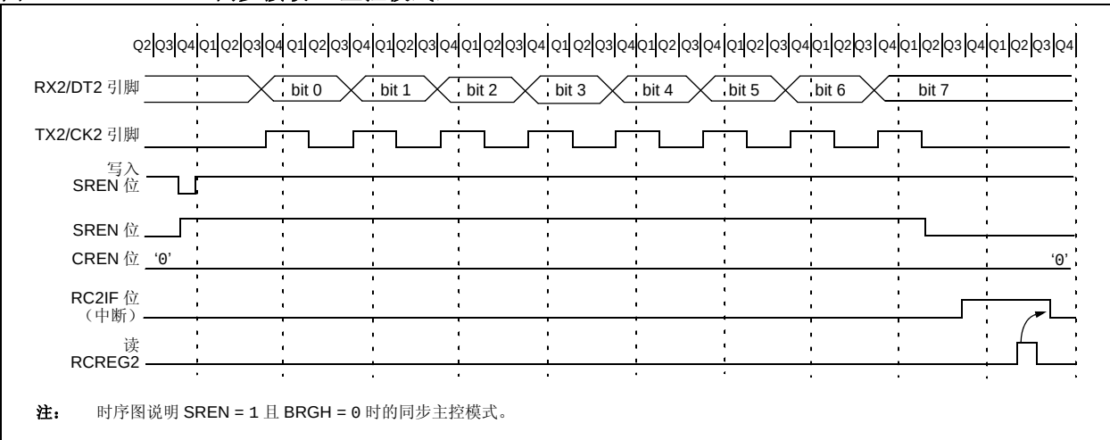
图 19-8: 同步接收（主控模式， SREN ）
