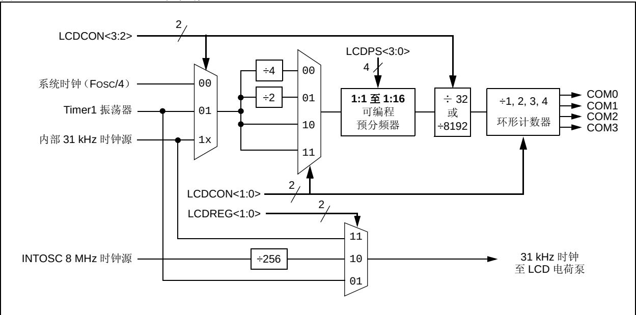
图 16-2: LCD 时钟的产生
