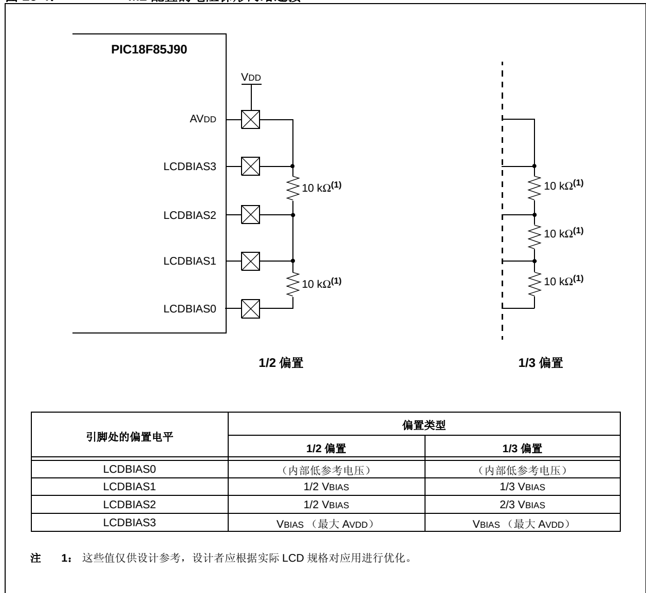
图 16-4: M2 配置的电阻梯形网络连接
