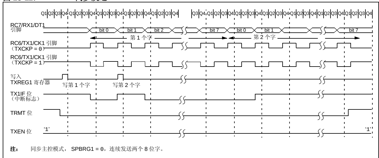
图 18-11: 同步发送
