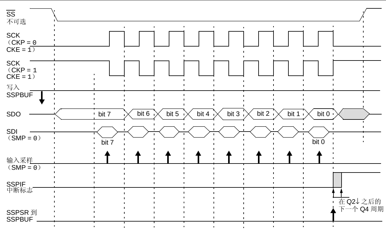
图 17-6: SPI 模式波形图 (从动模式, CKE = 1)
