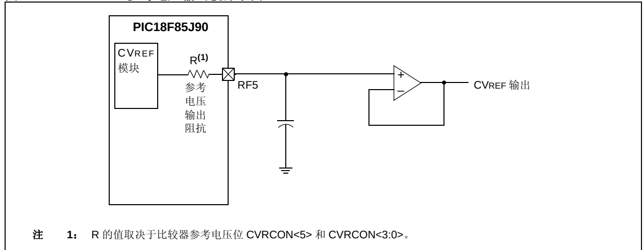
图 22-2: 参考电压输出缓冲示例
