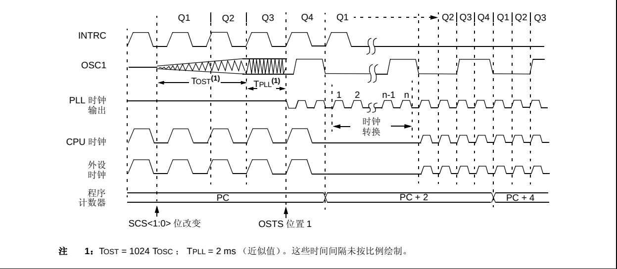
图 4-4: 从 RC_RUN 模式切换到 PRI_RUN 模式的转换时序
