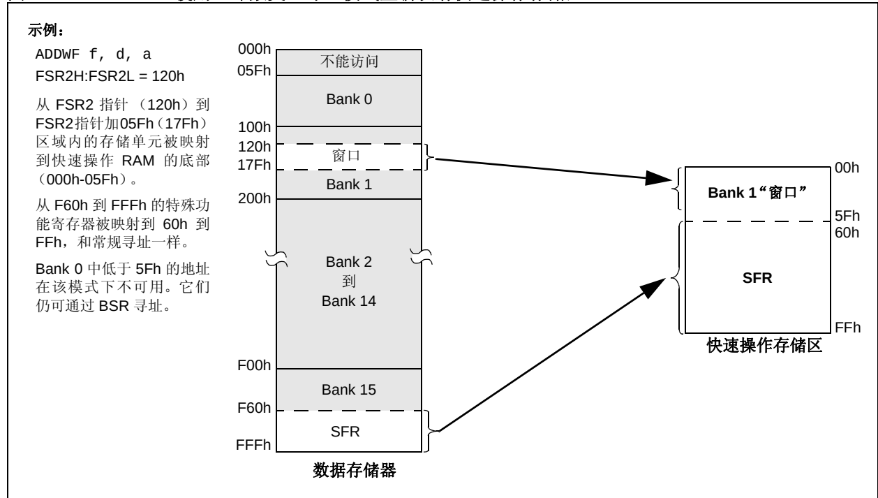
图 6-11: 使用立即数变址寻址模式重新映射快速操作存储区
