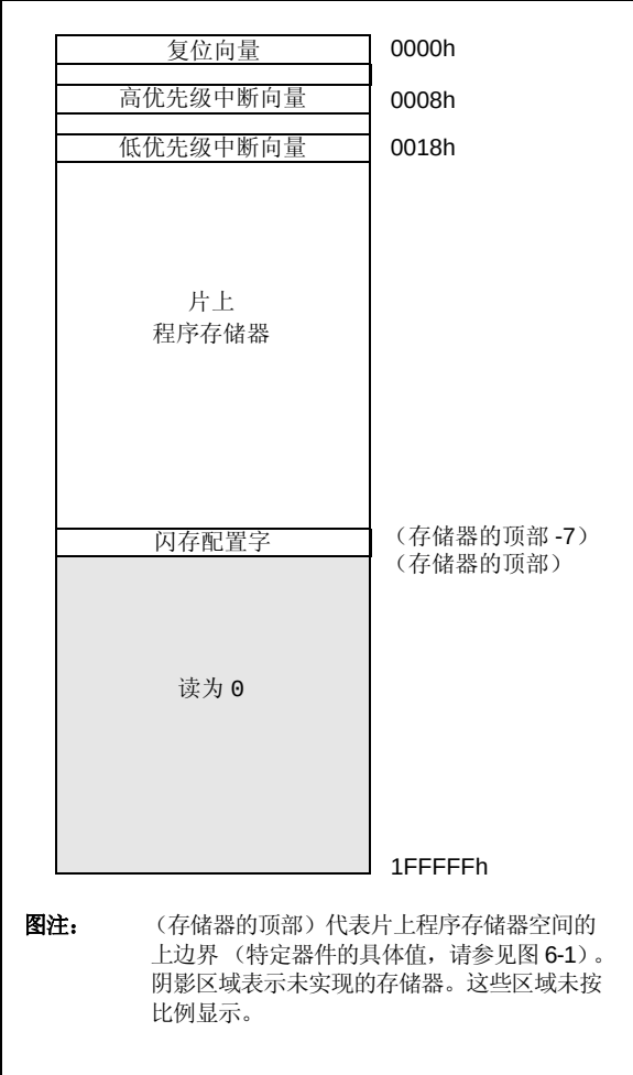
图 6-2: PIC18F85J90 系列器件的硬件编码向量和配置字单元
