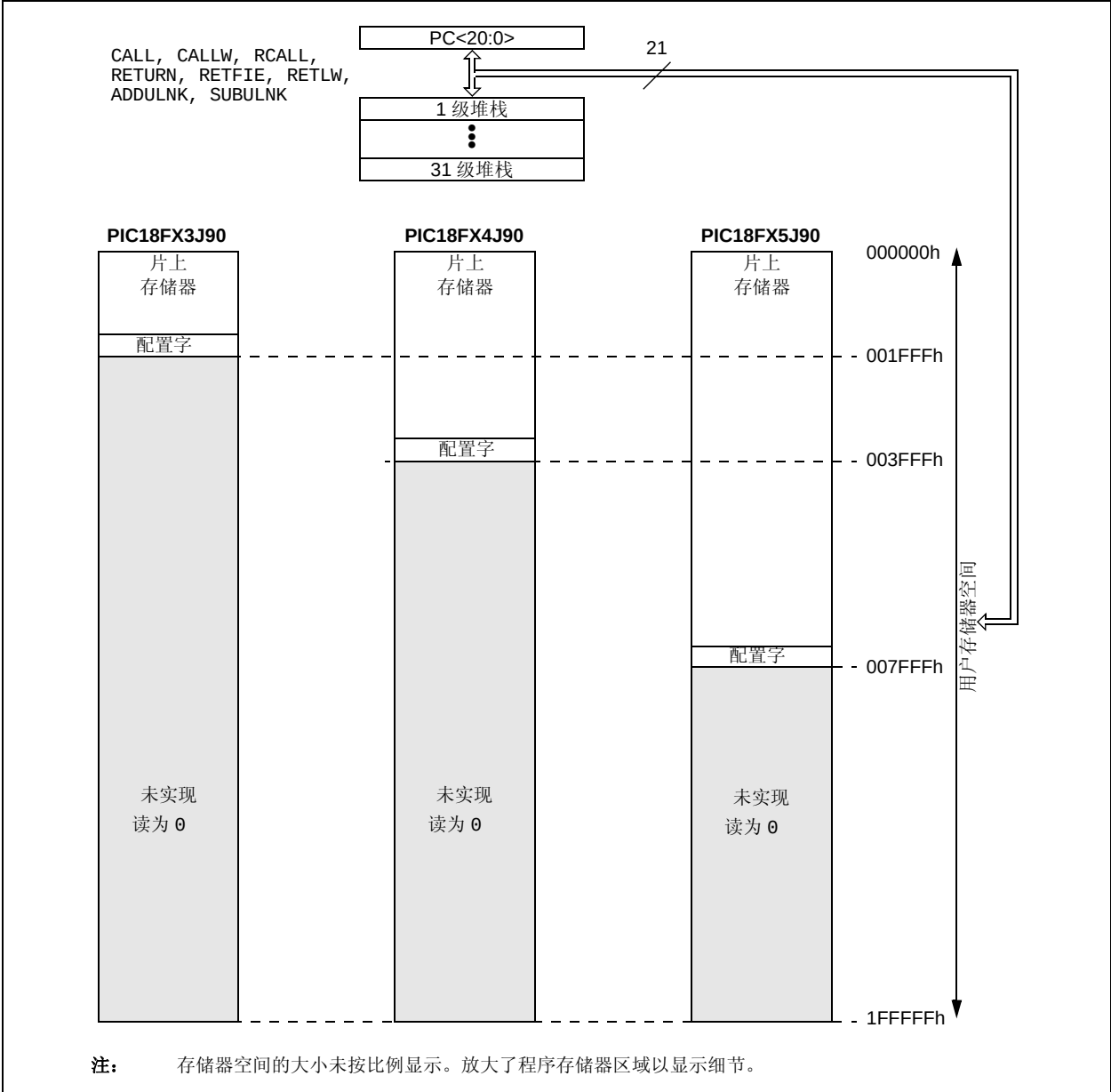
图 6-1: PIC18F85J90 系列器件的存储器映射图
