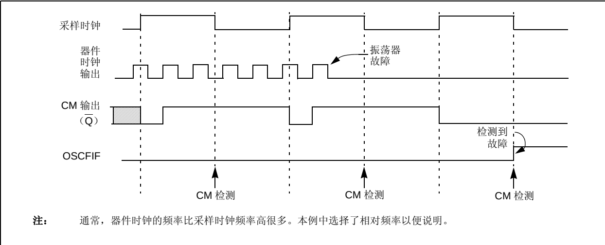
图 23-5: FSCM 时序图
