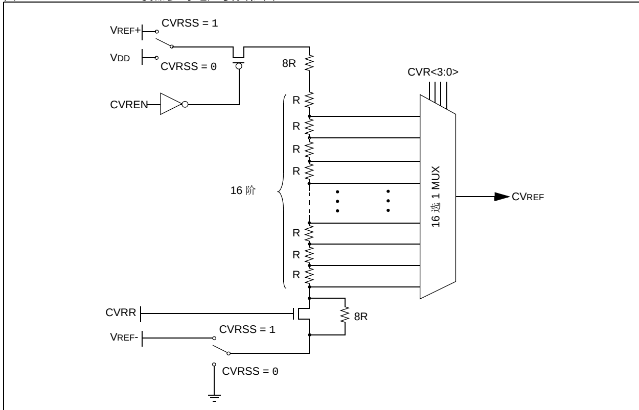
图 22-1: 比较器参考电压模块框图
