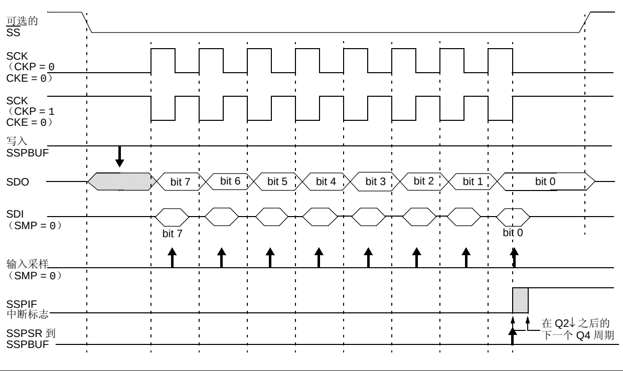
图 17-5: SPI 模式波形图 (从动模式, CKE = 0)
