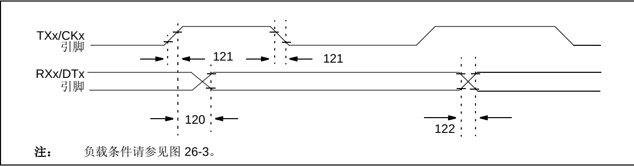
图 26-17: EUSART/AUSART 同步发送（主控 / 从动）时序
