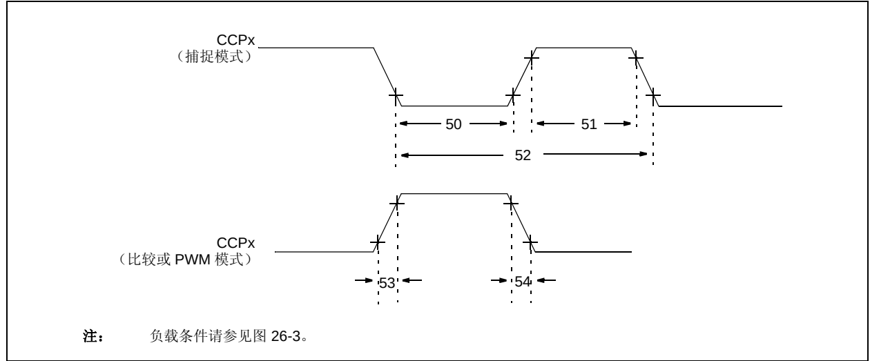
图 26-8: 捕捉 / 比较 / PWM 时序 (CCP1 和 CCP2 模块)
