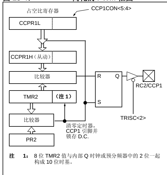
图 15-4: 简化的 PWM 框图
