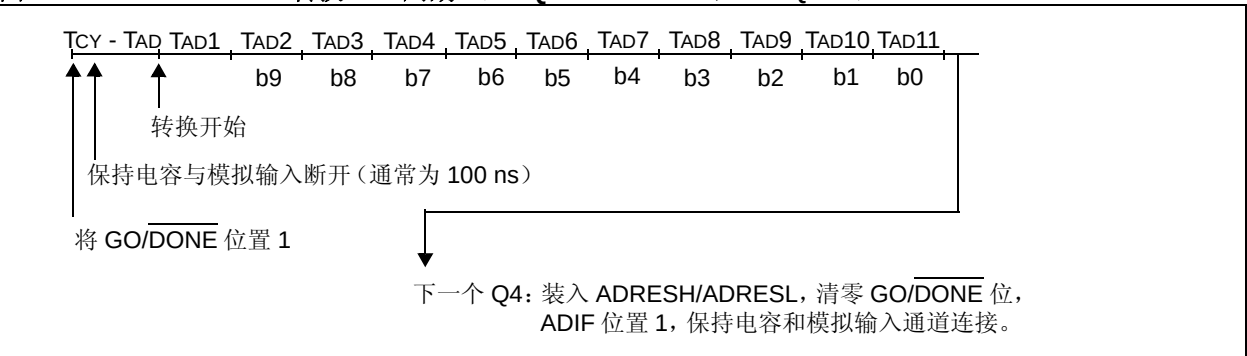
图 20-3: A/D 转换 TAD 周期 ( \text{ACQT}<2:0> = 000 , \text{TACQ} = 0 )
