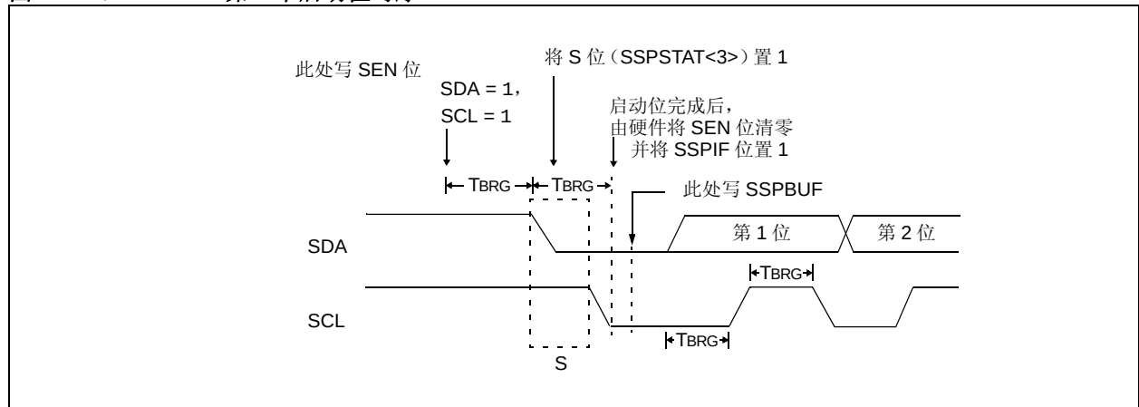
图 17-21: 第一个启动位时序
