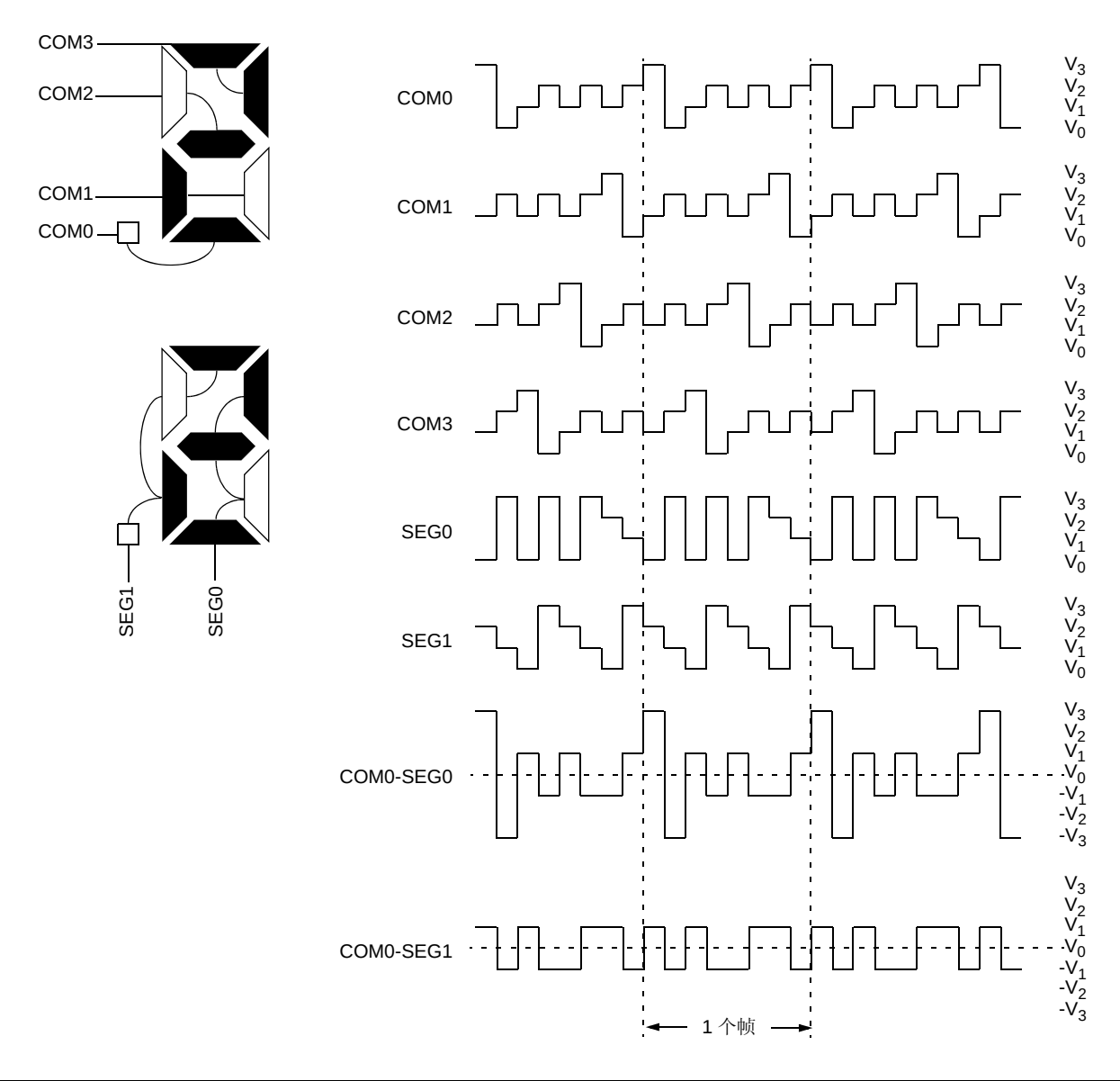
图 16-15: 在 1/4 复用、1/3 偏置驱动时的 A 型波形
