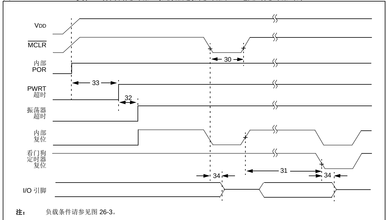
图 26-6: 复位、看门狗定时器、振荡器起振定时器和上电延时定时器时序
