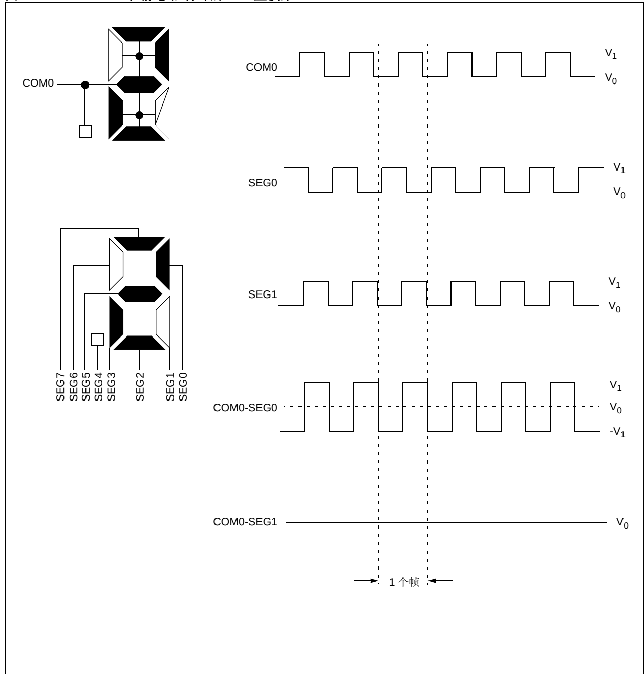
图 16-6: 在静态驱动时的 A/B 型波形
