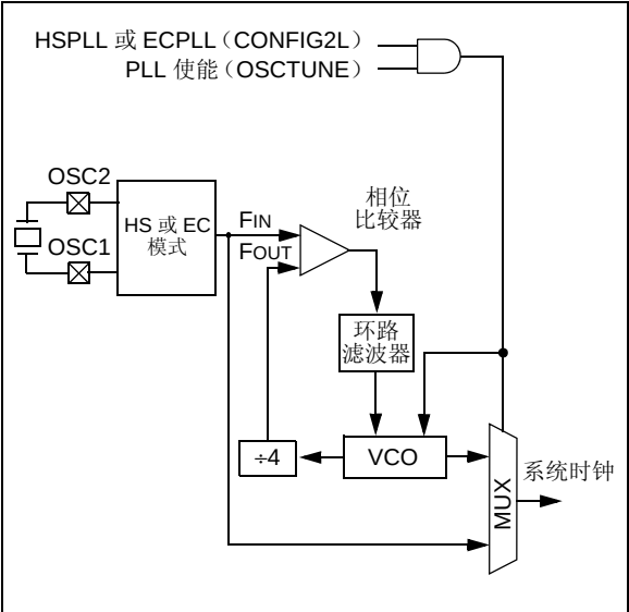
图 3-5: PLL 框图
