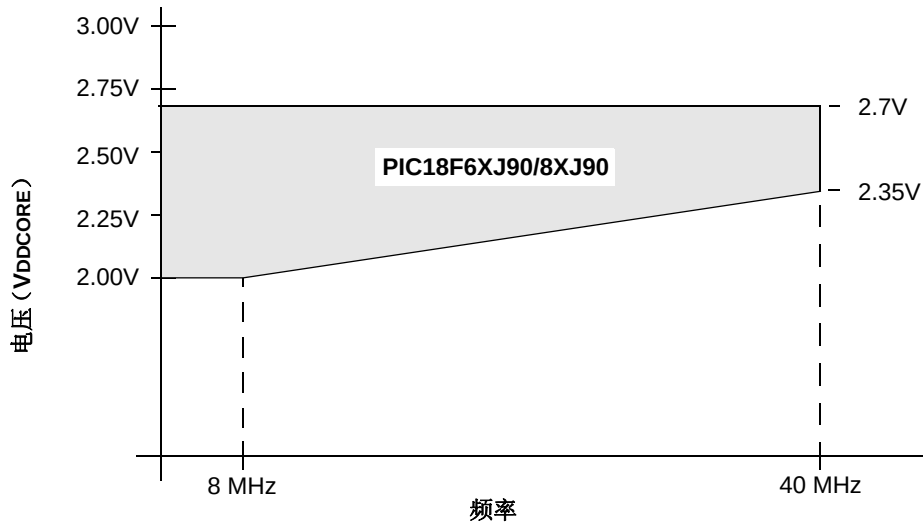
图 26-2: PIC18F85J90 系列电压—频率关系图，禁止稳压器（工业级） (1,2)
