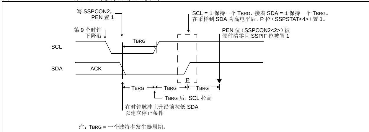
图 17-26: 停止条件接收或发送模式
