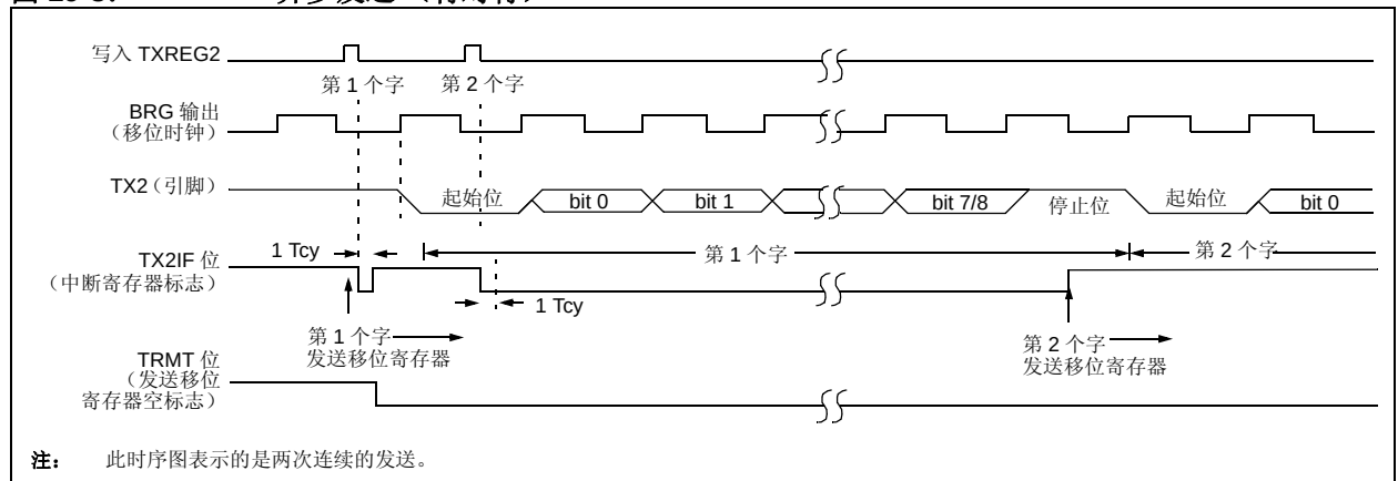
图 19-3: 异步发送（背对背）
