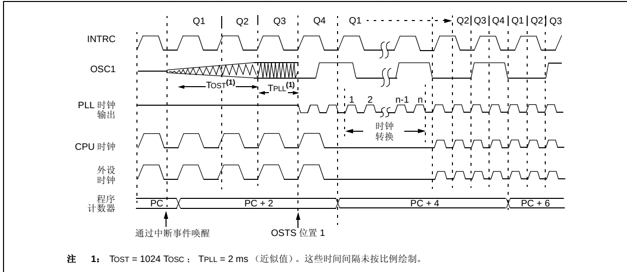
图 23-3: 双速启动时钟转换的时序图（从 INTRC 切换到 HSPLL）
