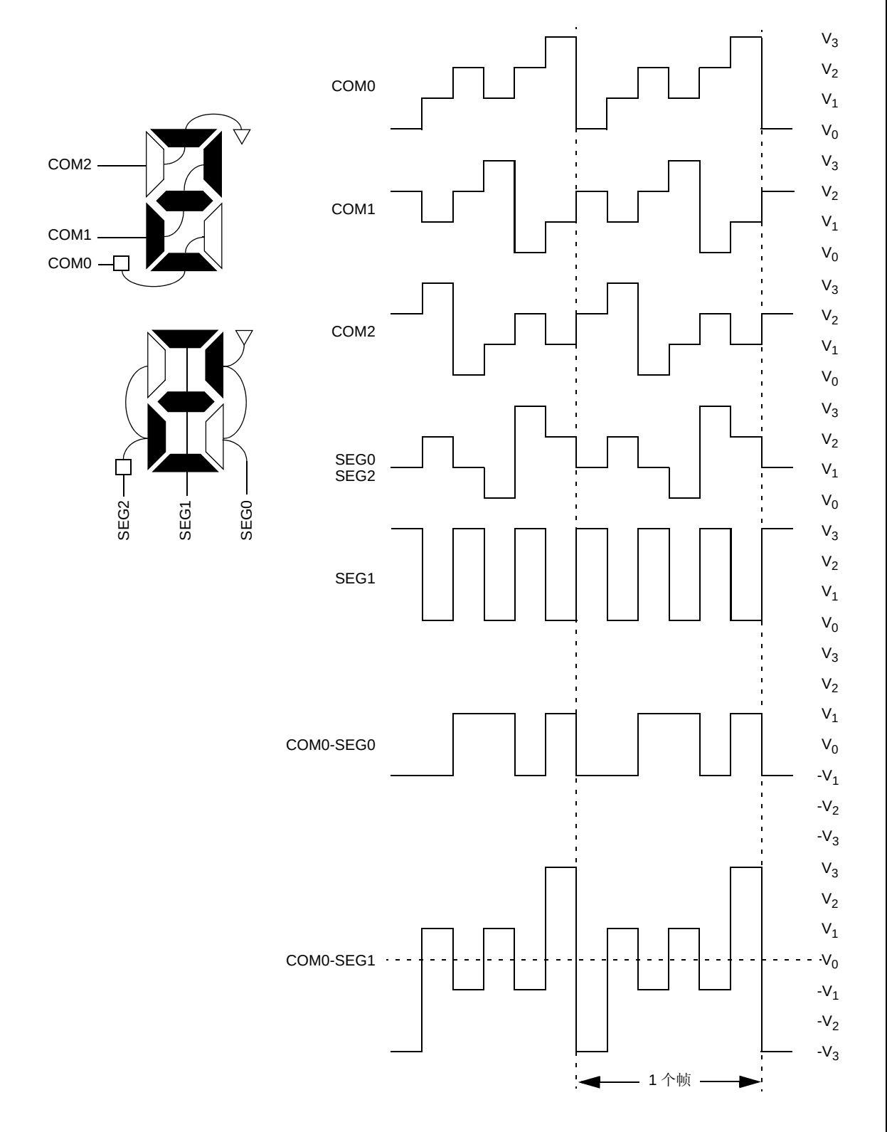
图 16-13: 在 1/3 复用、1/3 偏置驱动时的 A 型波形
