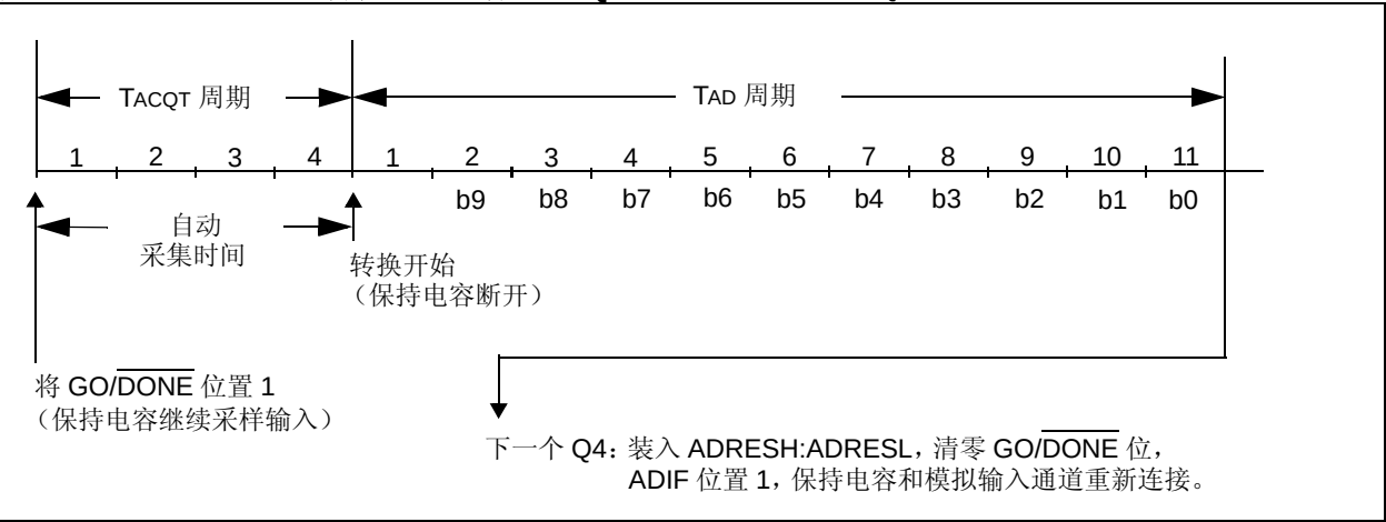
图 20-4: A/D 转换 TAD 周期 ( \text{ACQT}<2:0> = 010 , \text{TACQ} = 4 \text{ TAD} )
