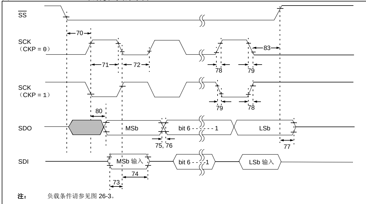
图 26-11: SPI 从动模式时序示例 (CKE = 0)
