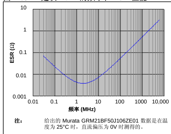
图 2-3: 建议 VCAP 的频率和 ESR 性能
