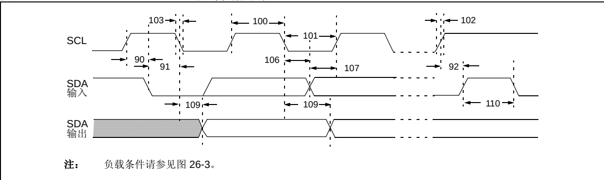
图 26-16: MSSP I 2 C™ 总线数据时序
