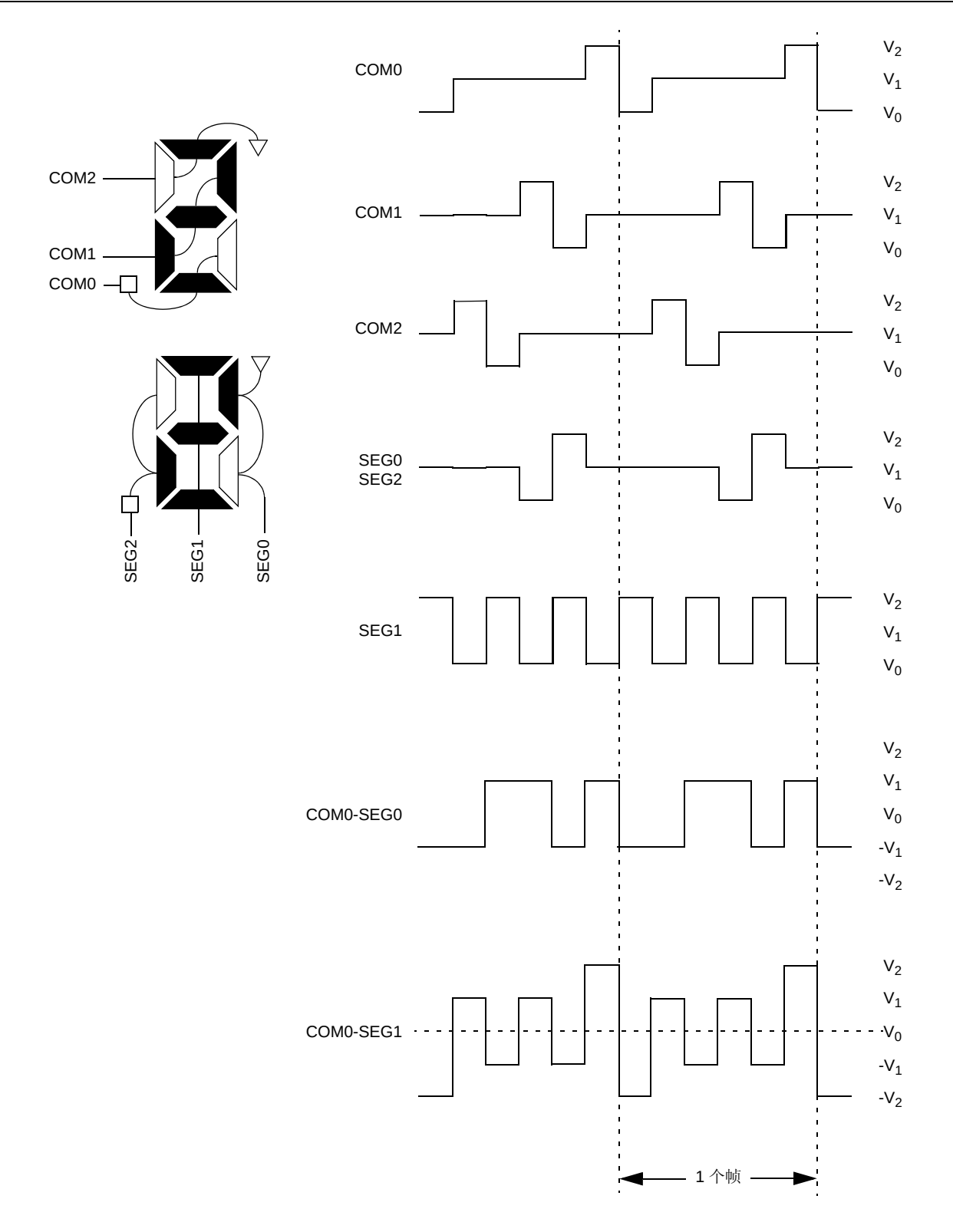
图 16-11: 在 1/3 复用、1/2 偏置驱动时的 A 型波形
