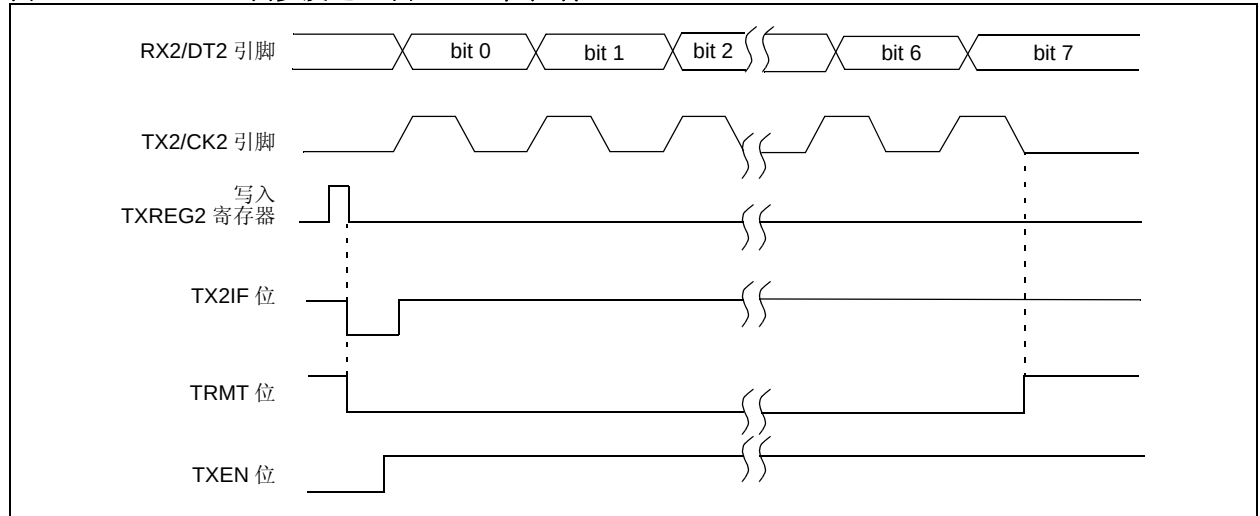
图 19-7: 同步发送（由 TXEN 位控制）
