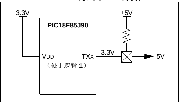
图 10-2: 使用漏极开路输出 (以 USART 为例)
