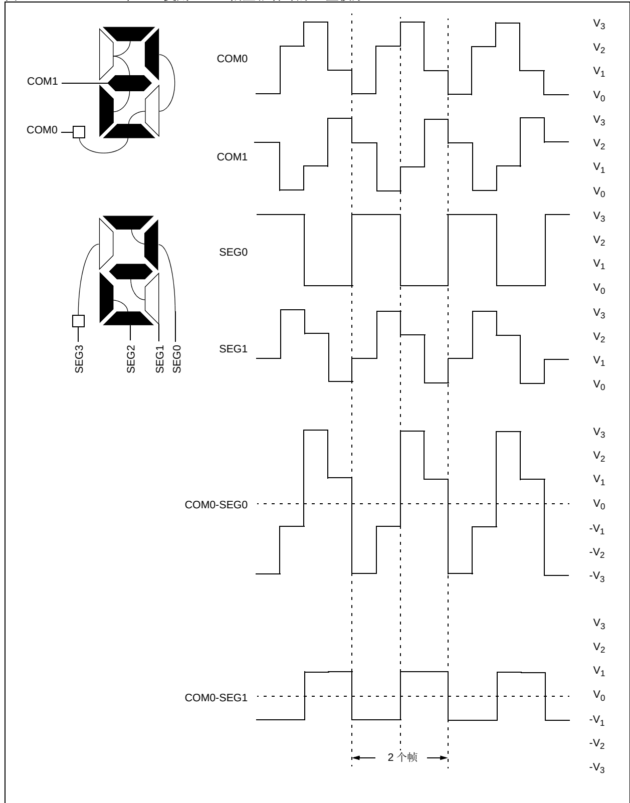
图 16-10: 在 1/2 复用、1/3 偏置驱动时的 B 型波形
