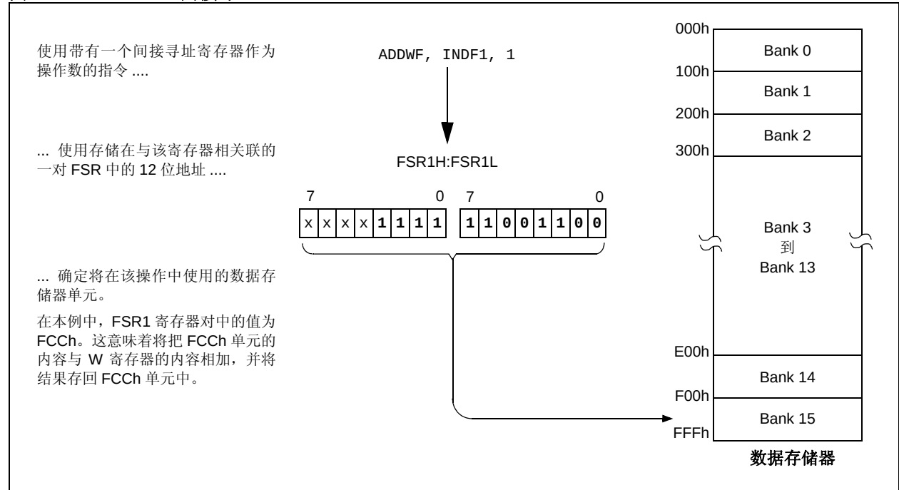
图 6-9: 间接寻址
