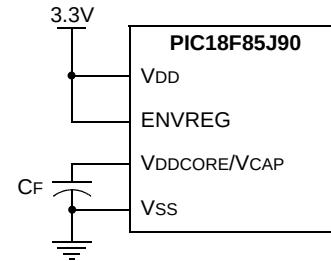
图 23-2: 片上稳压器连接
