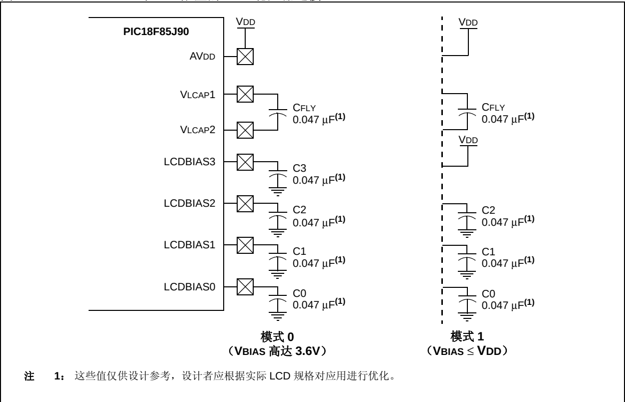
图 16-3: M0 和 M1 配置的 LCD 稳压器连接
