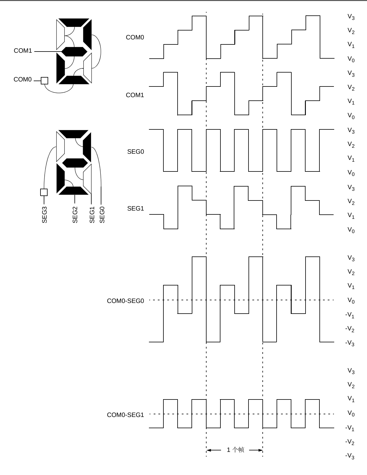
图 16-9: 在 1/2 复用、1/3 偏置驱动时的 A 型波形
