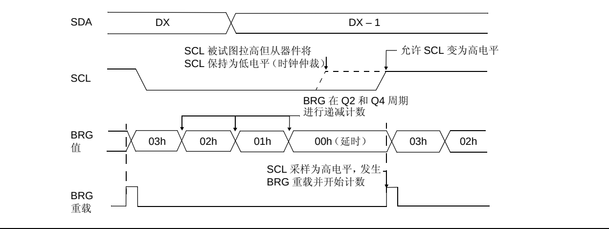
图 17-20: 带有时钟仲裁的波特率发生器时序
