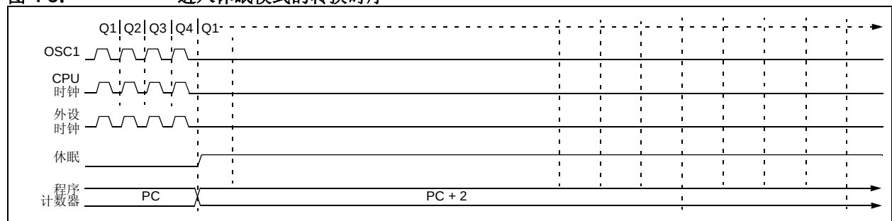
图 4-6: 从休眠模式唤醒的时序转换（HSPLL）
