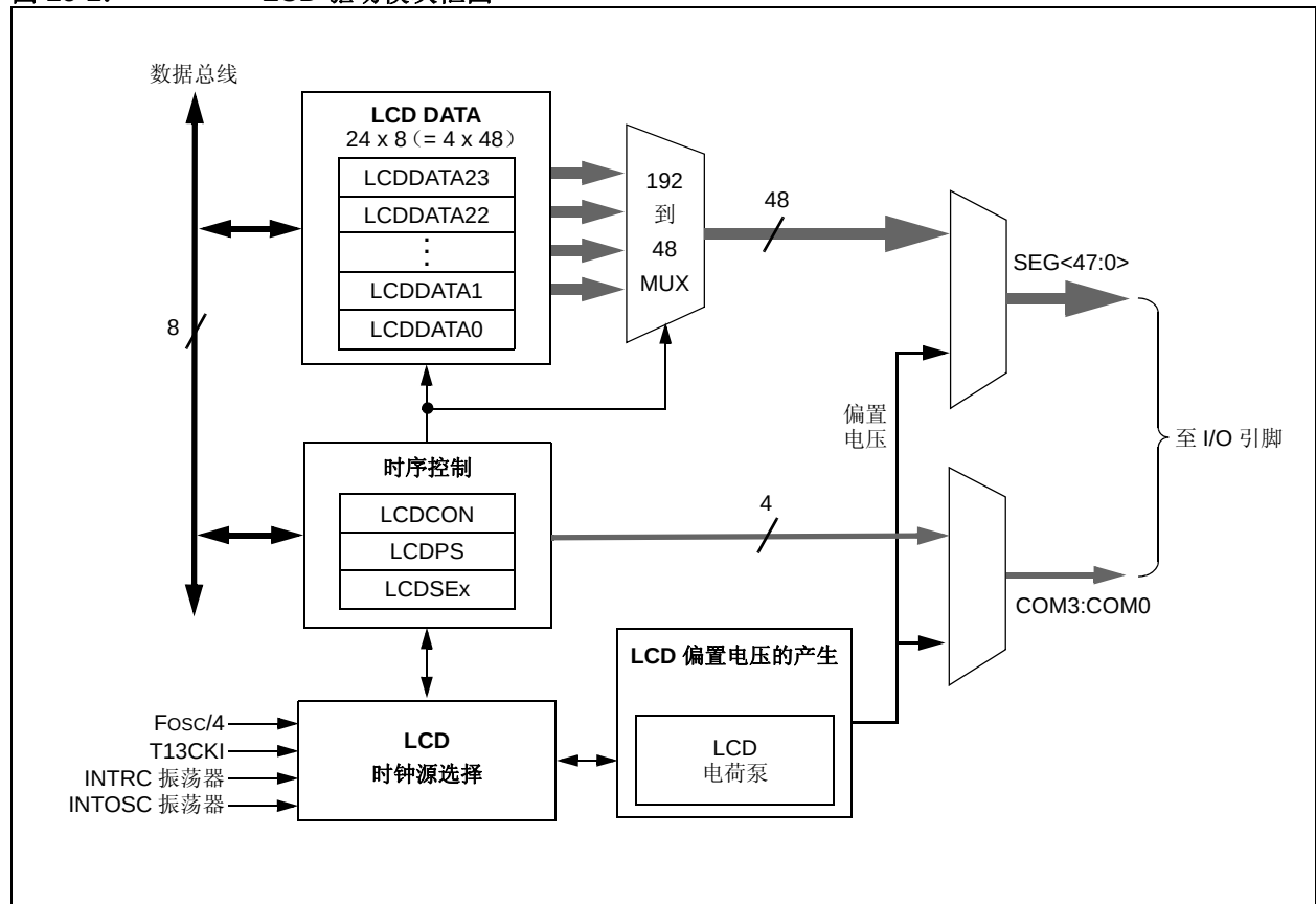
图 16-1: LCD 驱动模块框图
