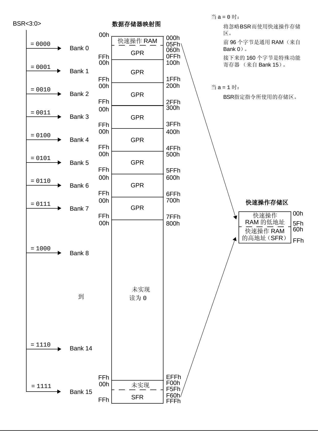
图 6-7: PIC18FX5J90 器件的数据存储器映射图
