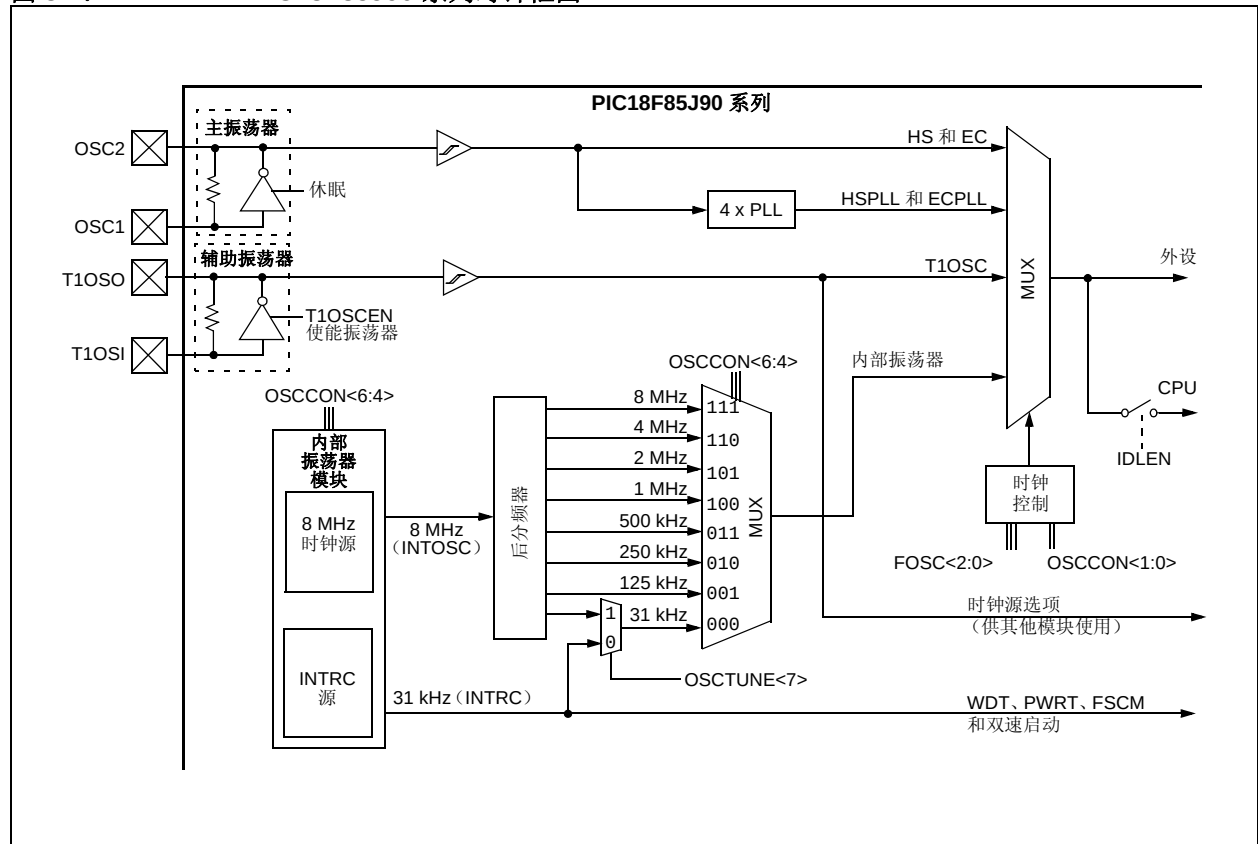
图 3-1: PIC18F85J90 系列时钟框图
