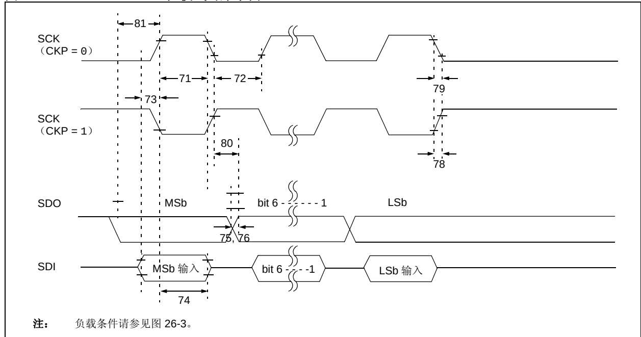
图 26-10: SPI 主控模式时序示例 (CKE = 1)
