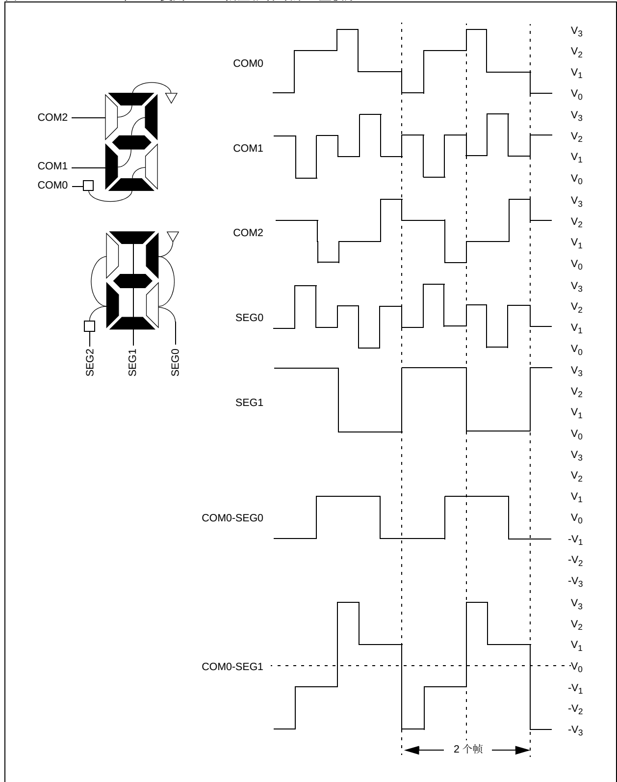
图 16-14: 在 1/3 复用、1/3 偏置驱动时的 B 型波形
