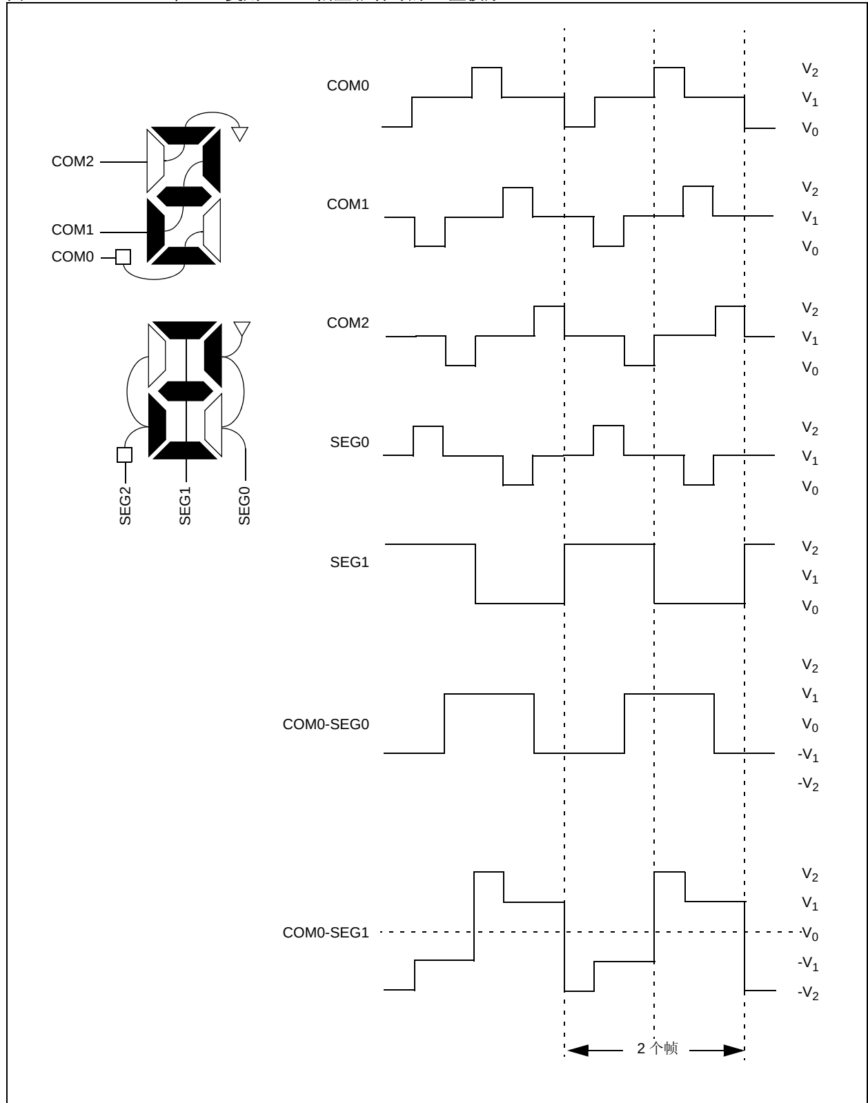
图 16-12: 在 1/3 复用、1/2 偏置驱动时的 B 型波形
