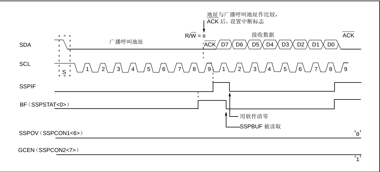
图 17-17: 从动模式广播呼叫地址序列（7 位或 10 位地址模式）
