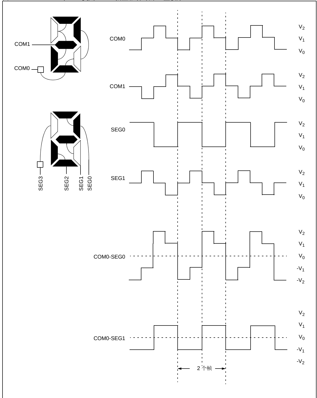
图 16-8: 在 1/2 复用、1/2 偏置驱动时的 B 型波形
