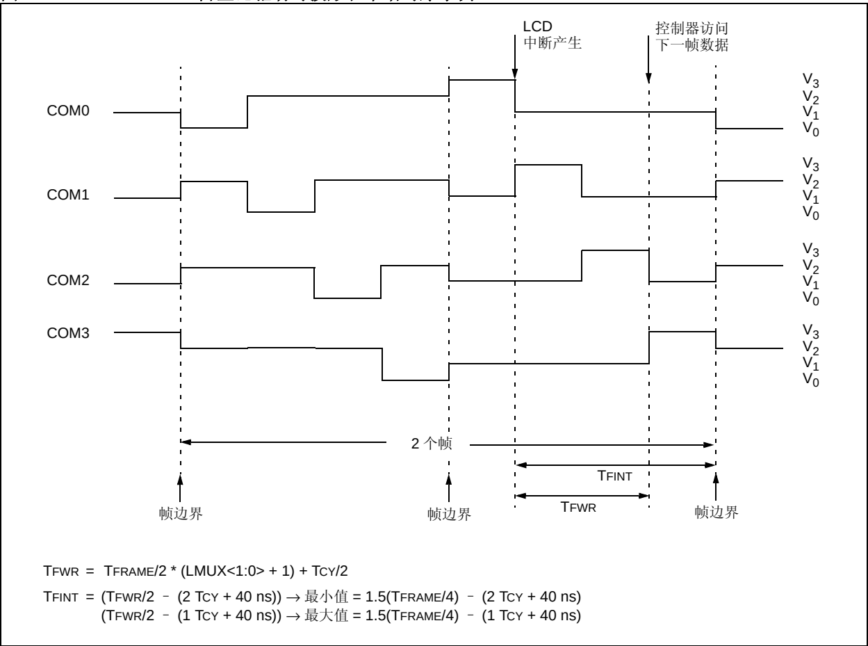
图 16-17: 1/4 占空比驱动时波形和中断时序示例
