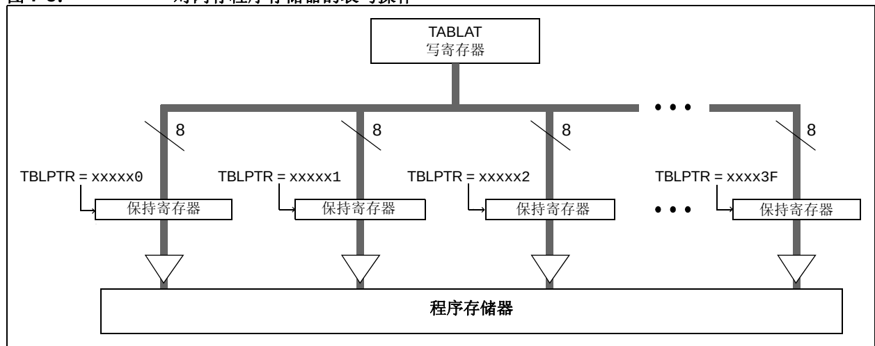
图 7-5: 对闪存程序存储器的表写操作
