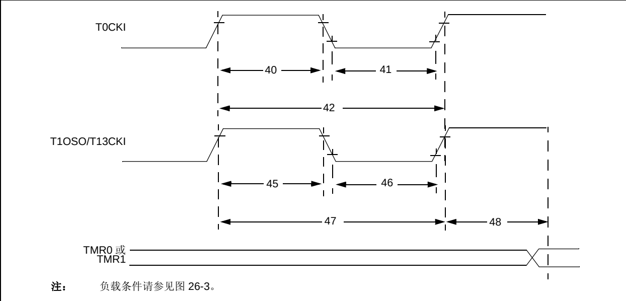
图 26-7: TIMER0 和 TIMER1 外部时钟时序
