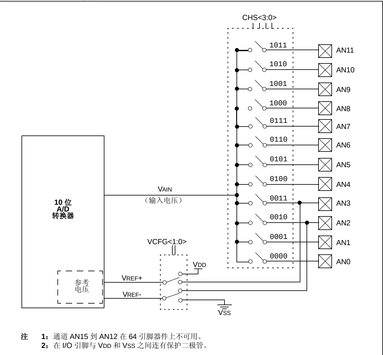
图 20-1: A/D 框图 (1,2)
