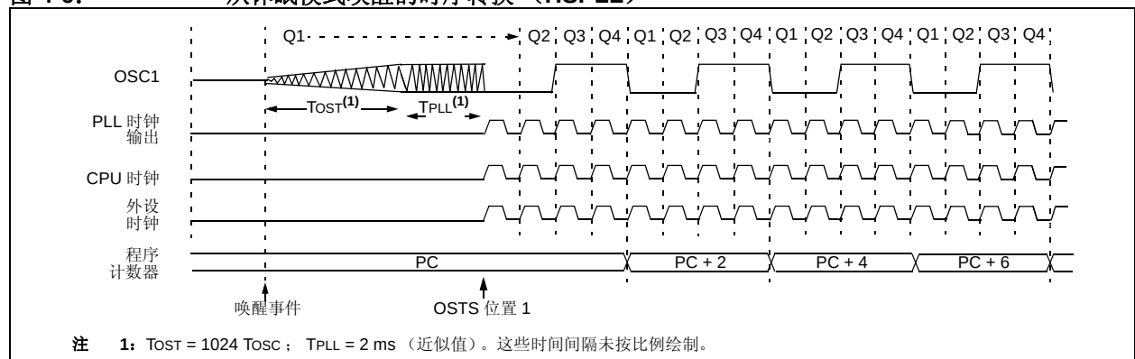
图 4-6: 从休眠模式唤醒的时序转换（HSPLL）
