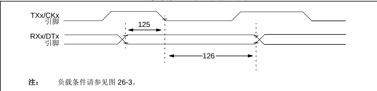
图 26-18: EUSART/AUSART 同步接收（主控 / 从动）时序
