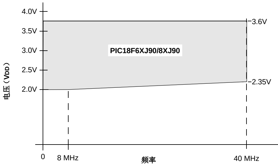
图 26-1: PIC18F85J90 系列电压—频率关系图，使能稳压器（工业级） (1)
