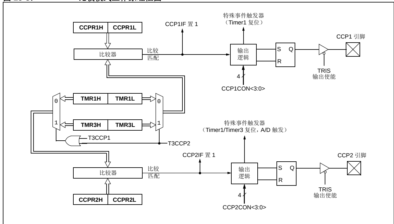
图 15-3: 比较模式工作原理框图
