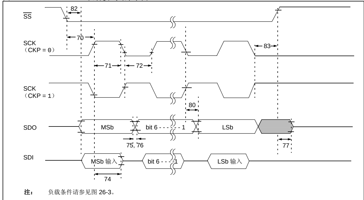
图 26-12: SPI 从动模式时序示例 (CKE = 1)
