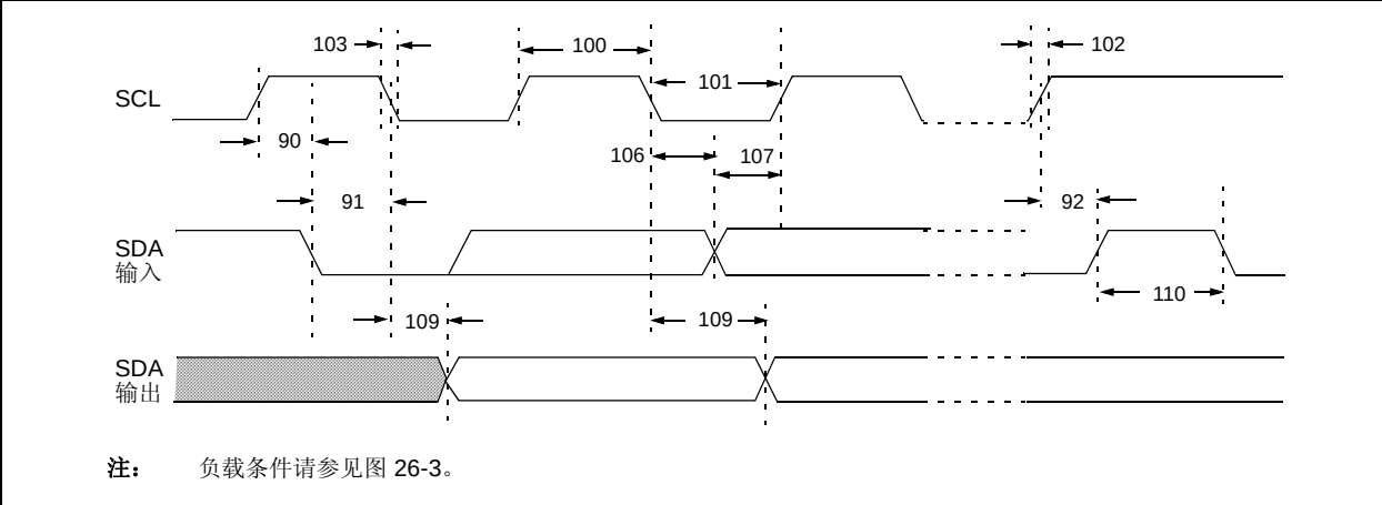
图 26-14: I 2 C™ 总线数据时序
