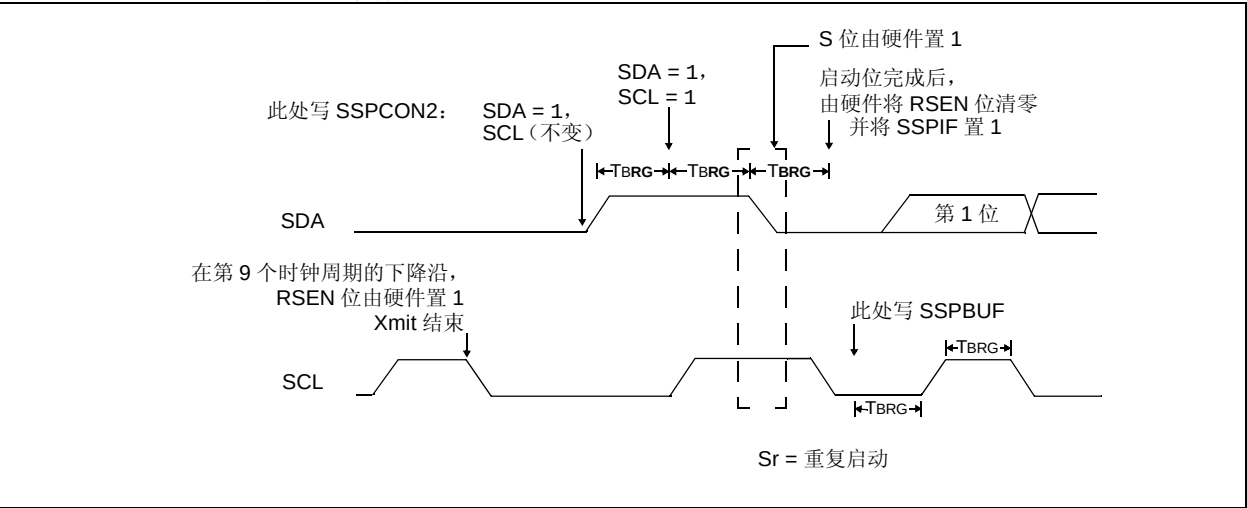
图 17-22: 重复启动条件波形图
