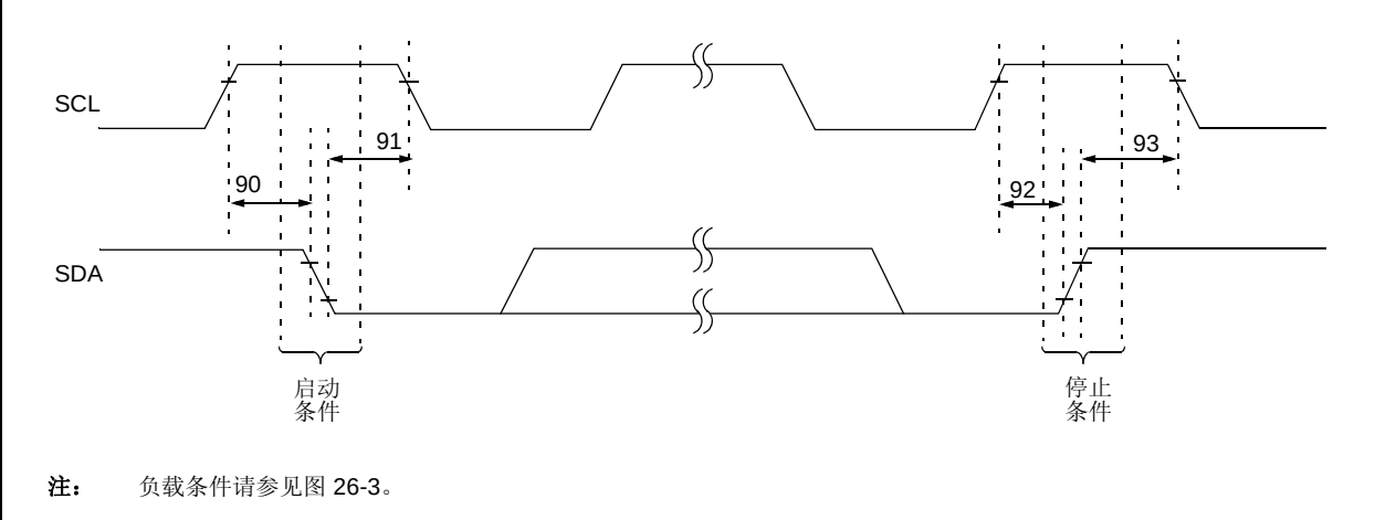
图 26-13: I 2 C™ 总线启动 / 停止位时序
