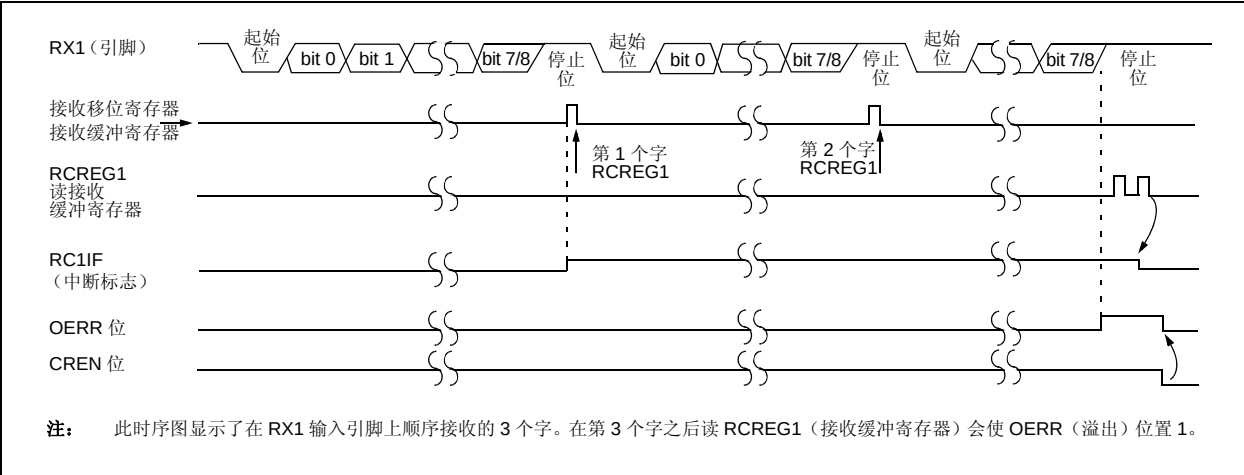
图 18-7: 异步接收
