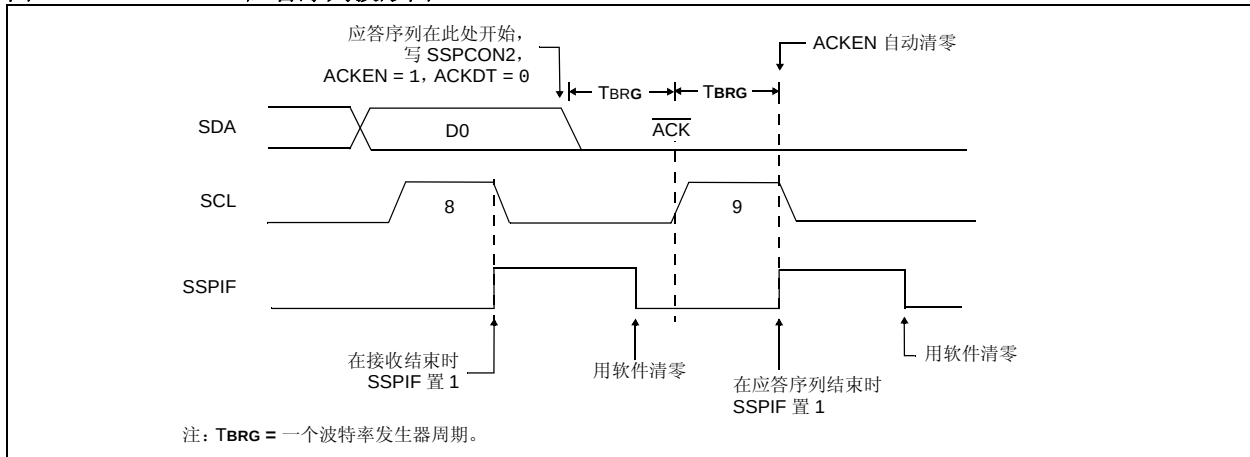
图 17-25: 应答序列波形图
