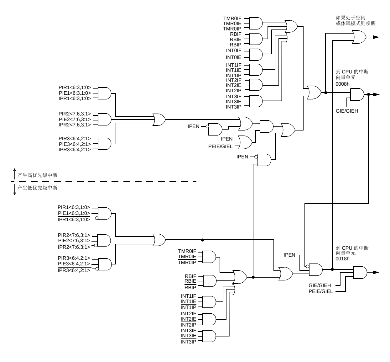
图 9-1: PIC18F85J90 系列中断逻辑
