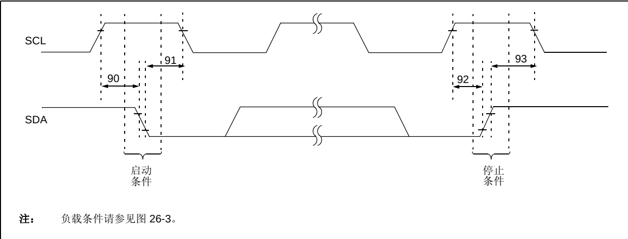
图 26-15: MSSP I 2 C™ 总线启动 / 停止位时序波形
