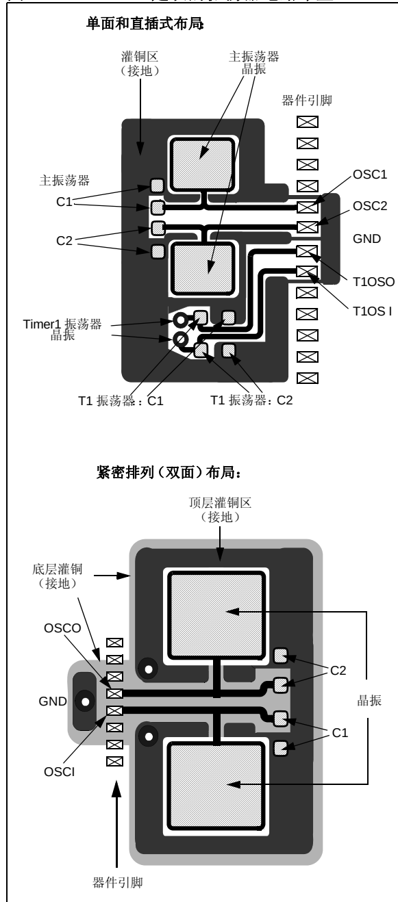
图 2-4: 建议的振荡器电路布置
