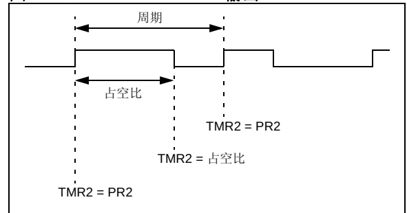
图 15-5: PWM 输出
