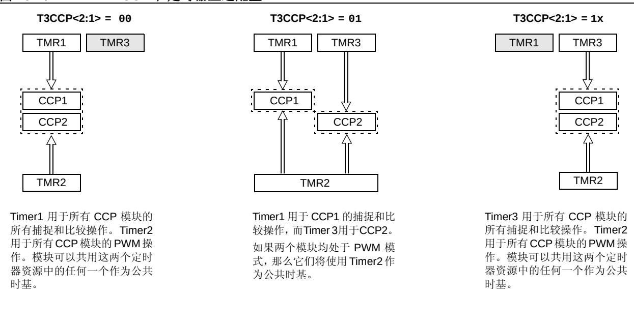
图 15-1: CCP 和定时器互连配置
