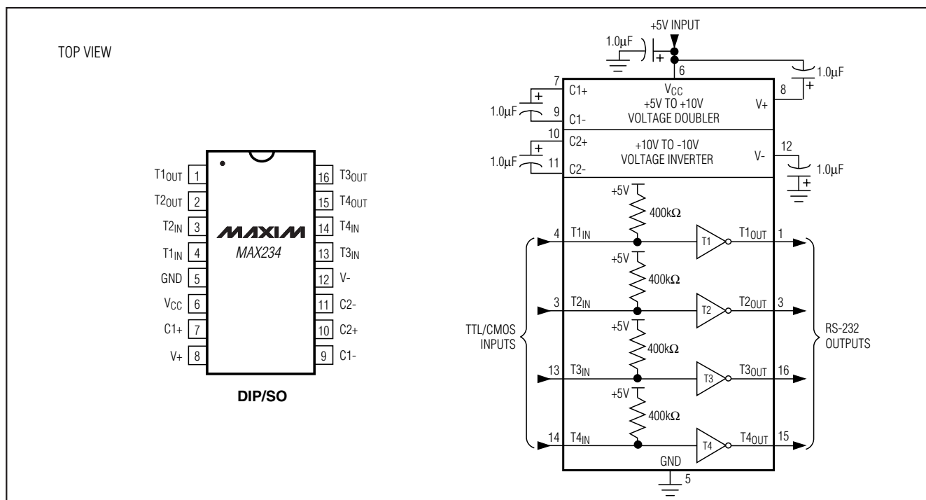
图 12. MAX234 引脚配置与典型工作电路
