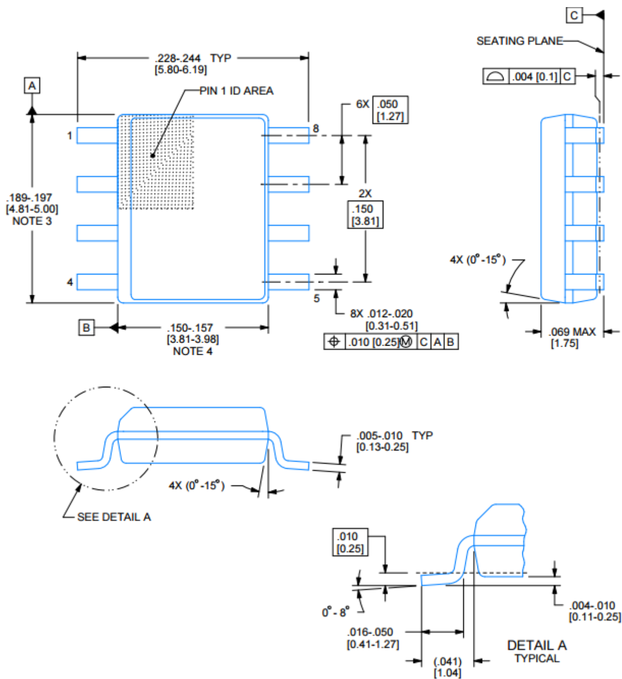
SOP8封装图
