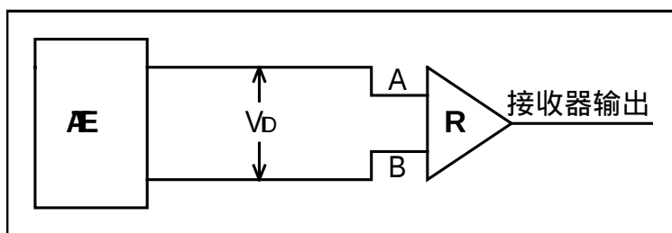
图 9: 接收器传输延时测试电路
