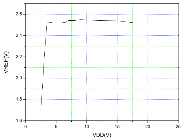
基准输出 vs. 工作电压
