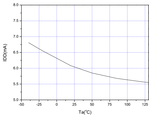
静态电流 vs. 温度
