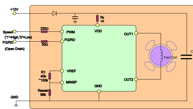
4 线 PWM 散热风扇(带最低转速设定)
