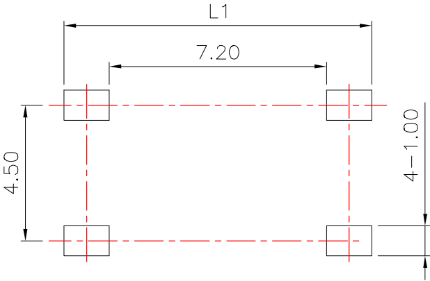
PCB Lavout(Pattern side)
