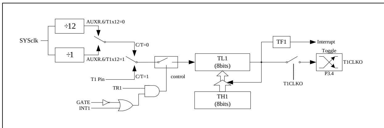
定时器/计数器 1 的模式 2: 8 位自动重装模式
