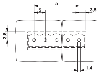
钻孔图
