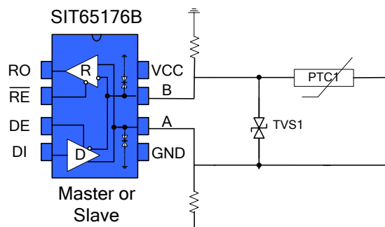
图 11 端口防护方案
