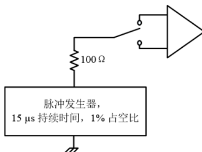
图 9 过压保护
