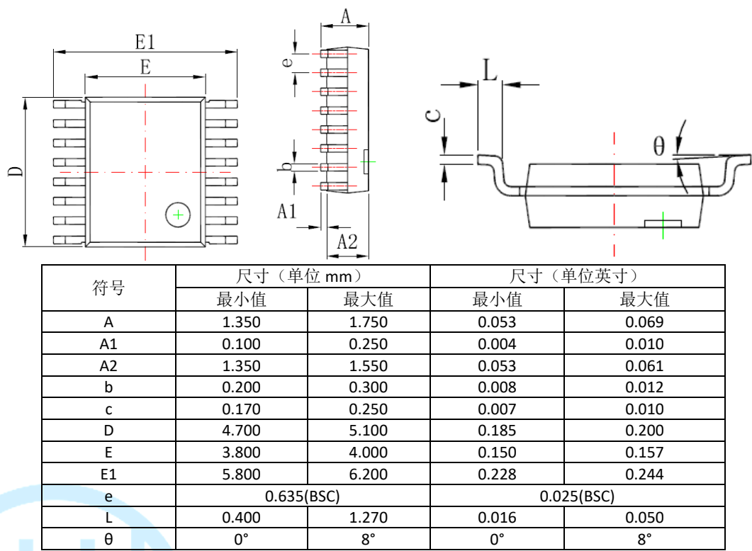
图 16. SSOP-16 封装外形尺寸
