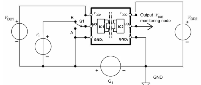
图 13.共模瞬变抗扰度(CMTI)测量
