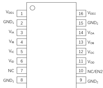
图 3. \pi 140U_{xx} 管脚定义
