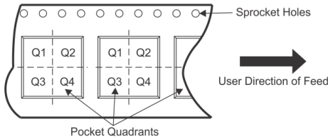
说明：芯片第一脚在象限 Q1。 图 22. 16 引脚宽体 SOIC 封装 [WB SOIC-16] 包装信息
