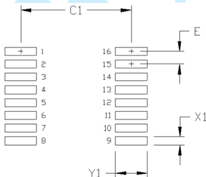
图 19. 16 引脚 SSOP 封装 [16-Lead SSOP] 焊盘图案
