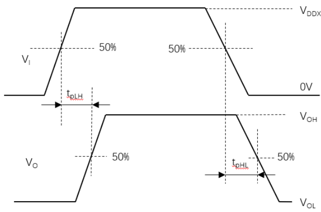
图 11.传输延迟时间波形测量
