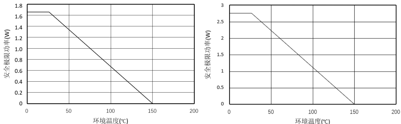
图 6.热降额曲线, 依据 DIN V VDE V 0884-11 的安全限值与环境温度的关系(左: \pi 14\text{xU}3\text{x} ; 右: \pi 14\text{xU}6\text{x} )
