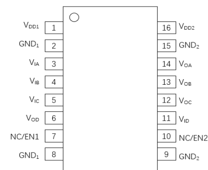
图 4. \pi 141U_{xx} 管脚定义
