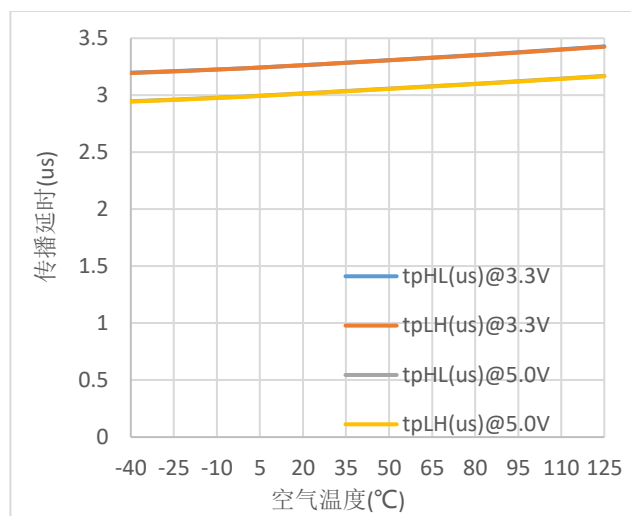
图 8.π14xU3x 传输延时 vs. 空气温度
