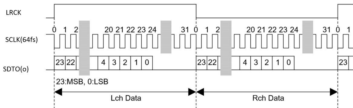
图 1. Mode 0 时序
