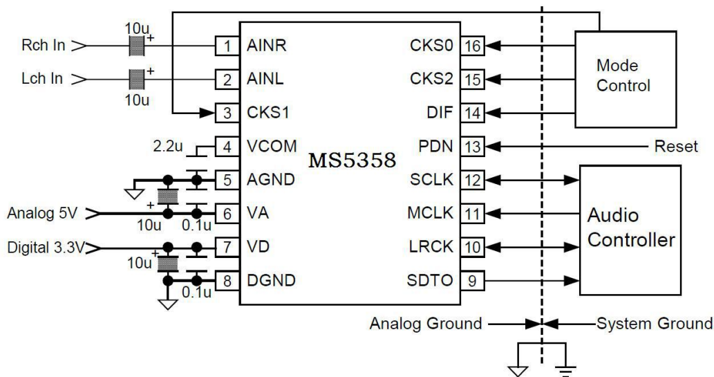
图 3. 典型连接图
