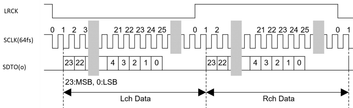
图 2. Mode 1 时序
