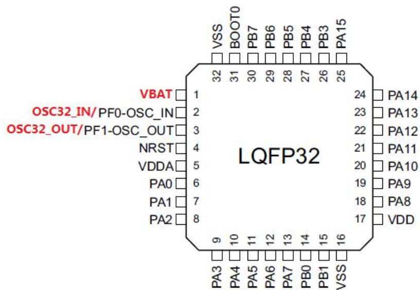
QFN32 封装 Pin-out
