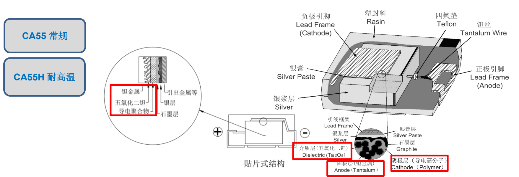
图 2. 片式导电聚合物钽电容器内部结构
