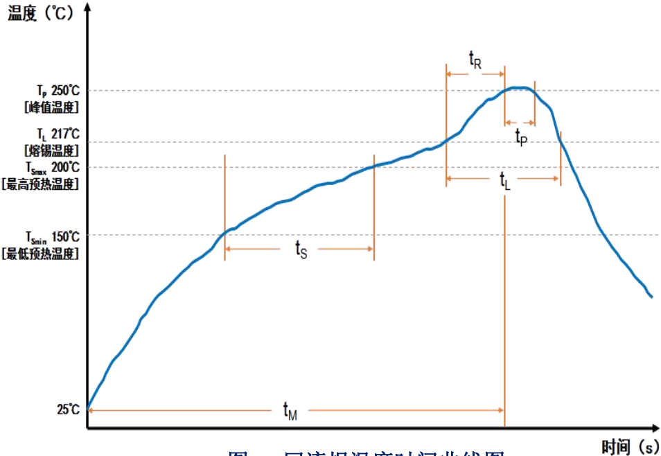
图 7. 回流焊温度时间曲线图
