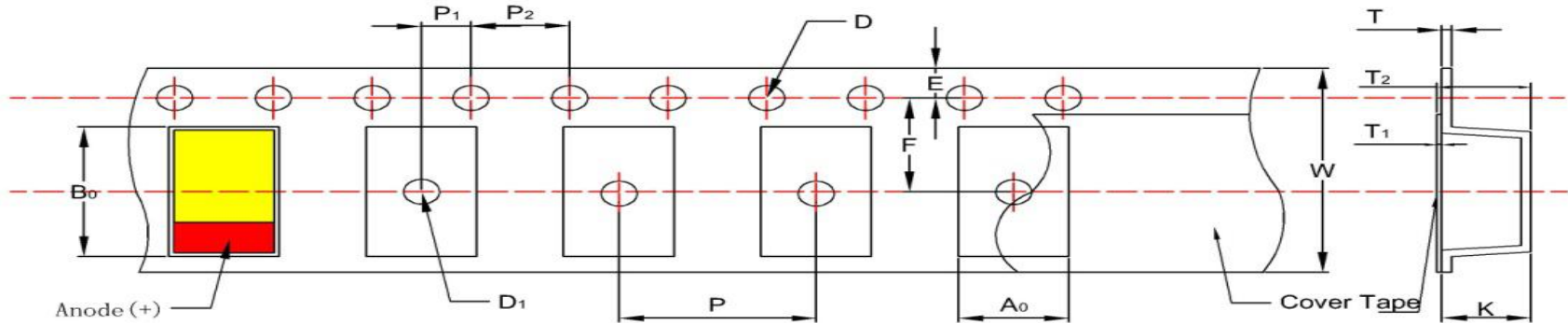
图 2 载带尺寸图
