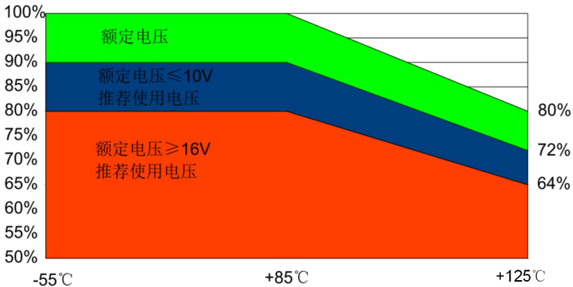
图 5. 高分子型产品工作电压
