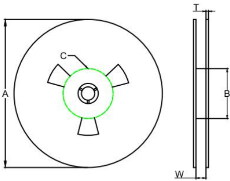
图 3 轮盘尺寸图
