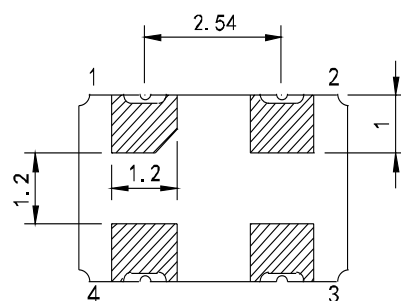
Bottom View 仰视图
