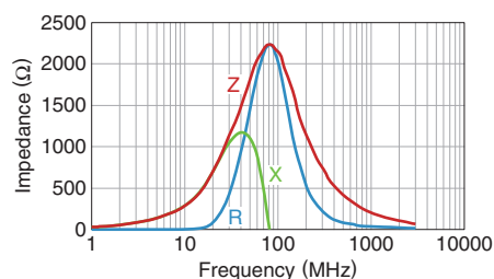
MMZ2012Y202BTD25
