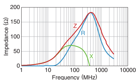
MMZ2012Y121BTD25
