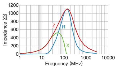
MMZ2012Y102BTD25
