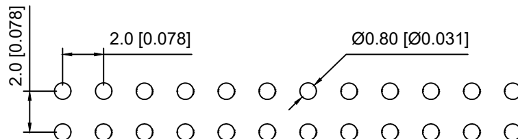
P.C.B LAYOUT
