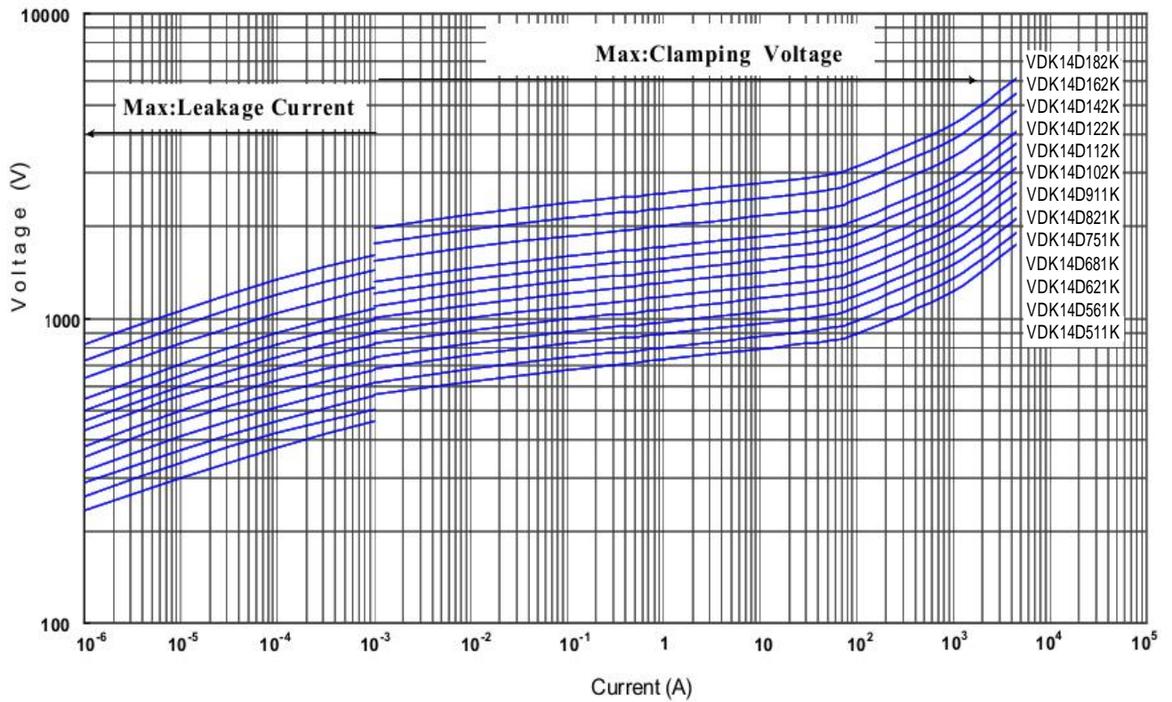
V-I Curve (VDK-14D511K to VDK-14D182K)
