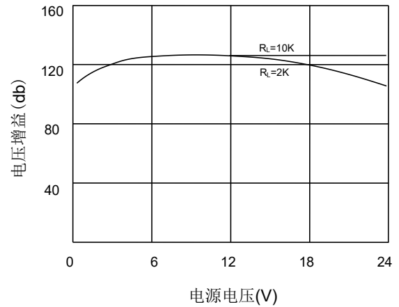
电压增益VS电源电压
