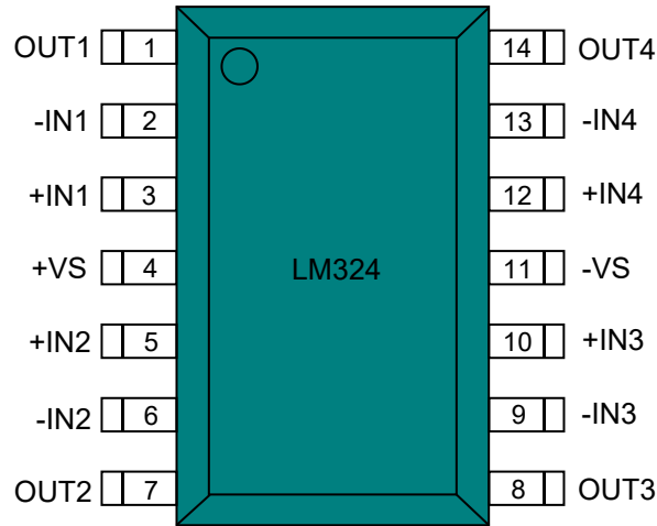
图2 LM324引脚定义图
