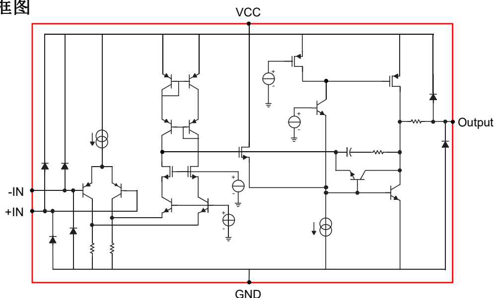
图1 LM324内部原理框图
