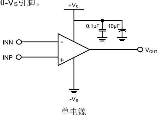
图5 电源旁路电容
