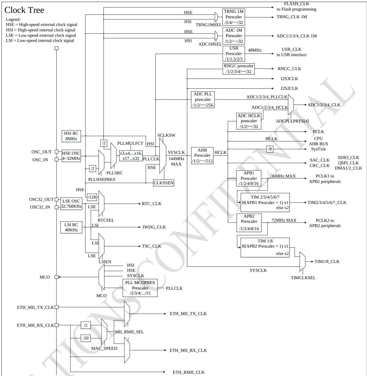
图 2-2 时钟树
