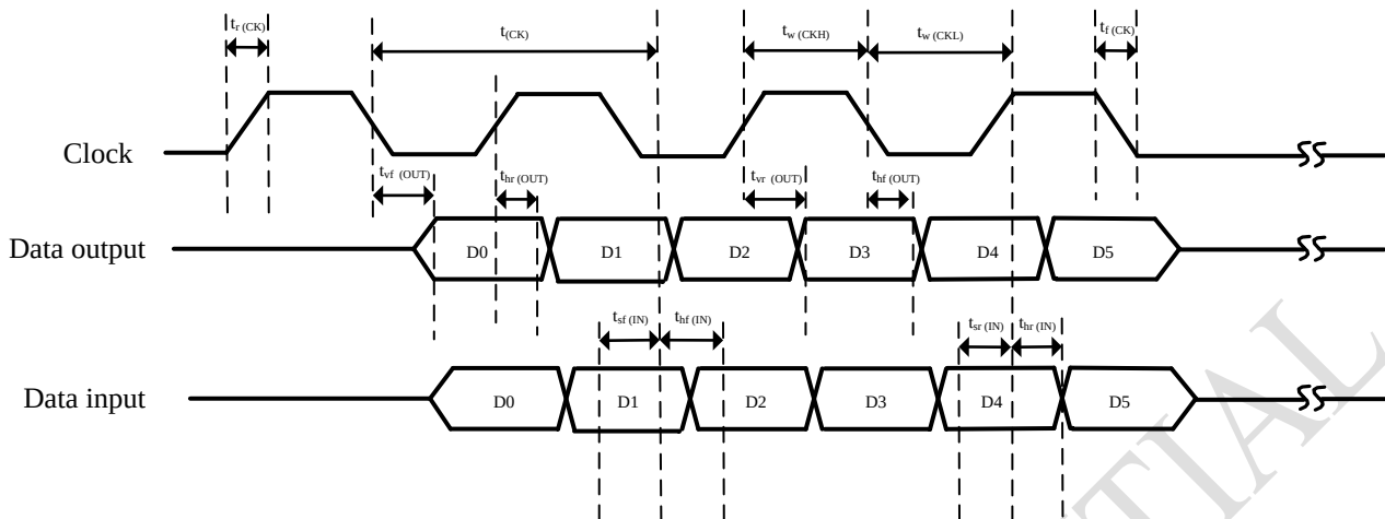
图 4-18 QSPI在DDR模式下的时序
