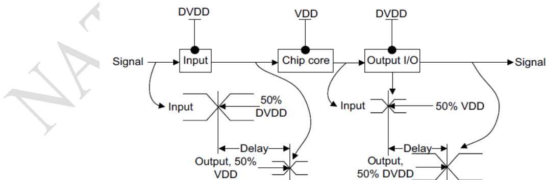
图 4-9 输入输出交流特性定义
