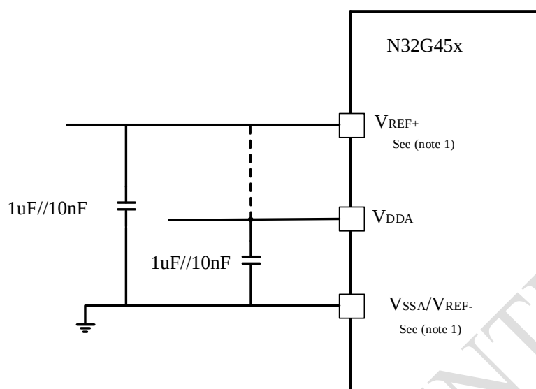
图 4-28 供电电源和参考电源去藕线路( V_{REF+} 未与 V_{DDA} 相连)
