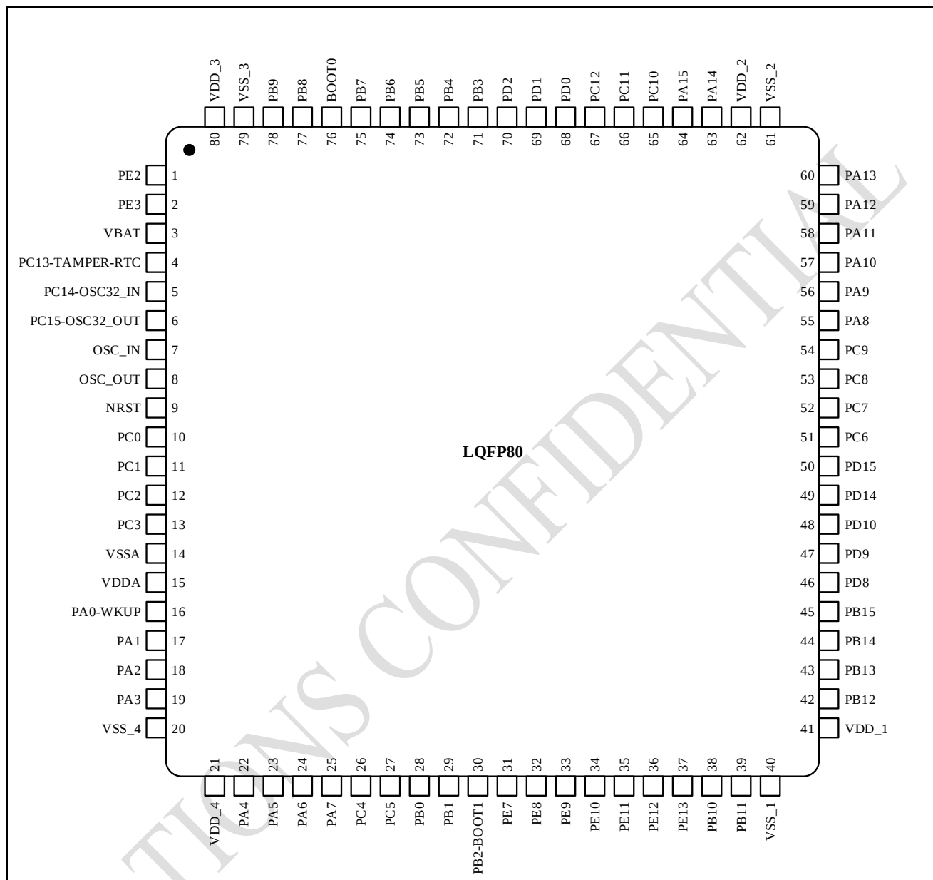
图 3-2 N32G457系列LQFP80引脚分布
