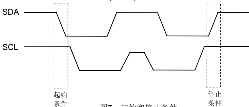
图7 起始和停止条件
