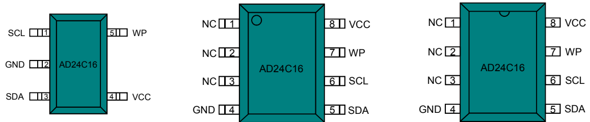
图2 AD24C16引脚定义图
