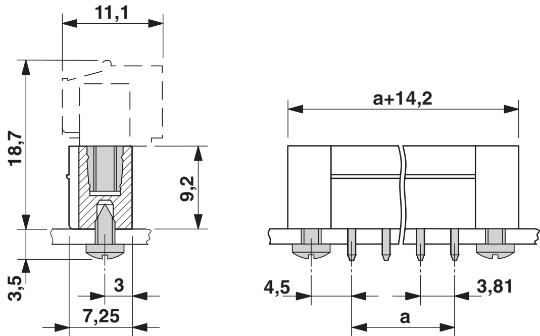
尺寸图
