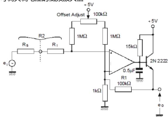
可调失调电压的低频放大器
