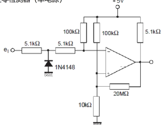
过零检测器 (单电源)
