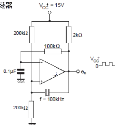
方波振荡器
