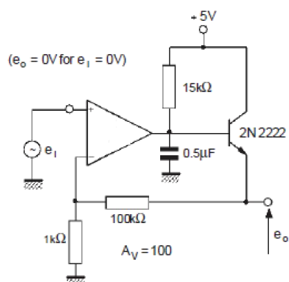
低频放大器
