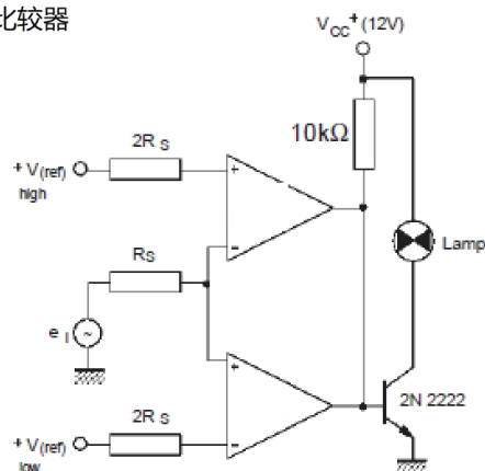
限幅比较器
