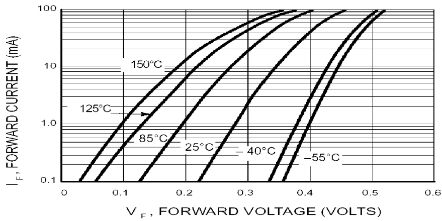
Fig.1 I_F — V_F
