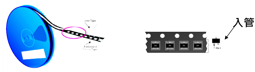
SOT-23 产品编带、包装图
