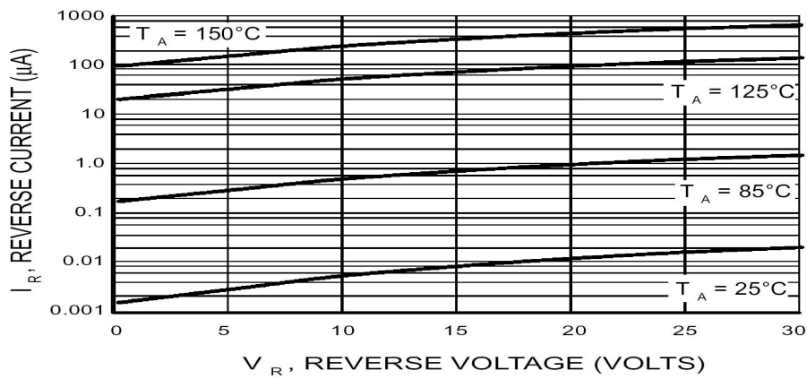
Fig.2 I_R — V_R
