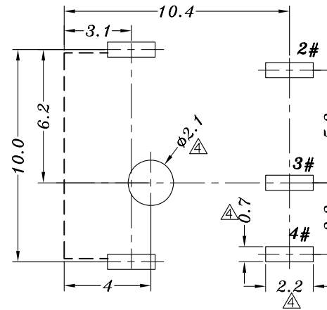
P.C.B LAYOUT
