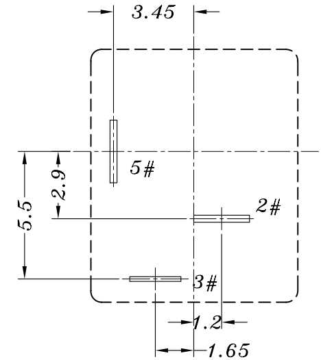
P.C.B LAYOUT
